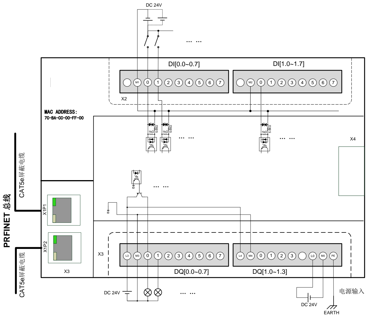
图 3 模块接线图
