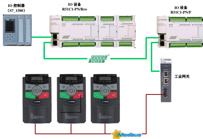
图 4:PROFINET IO 的网络结构
