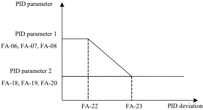
Figure 5-24. PID Parameter Switching
