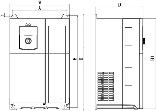
图 2-5. 380V (4T) 18~37kW 塑壳机箱外形尺寸及安装尺寸示意图
