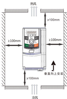
图3-1. 单体安装图
