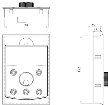
图2-14. 外引键盘带托盘安装尺寸图
