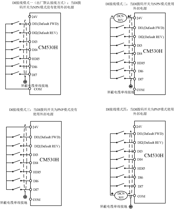
图3-10. 四种不同模式下数字输入端子接线图
