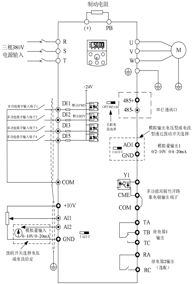
图 3-5.2. 2kW 以下三相变频器
