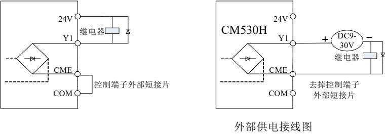
图3-11. 数字输出端子Y1接线示意图
