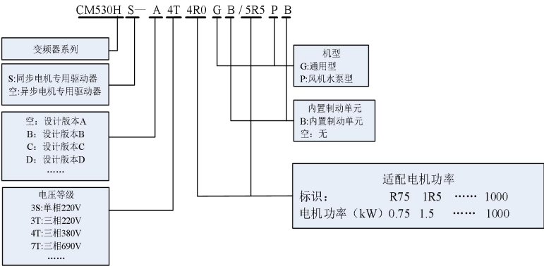
图2-1. 命名规格
