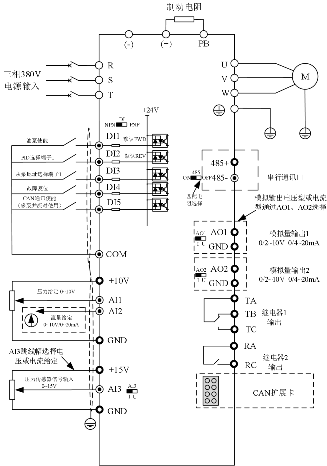
图 3-4. 接线图
