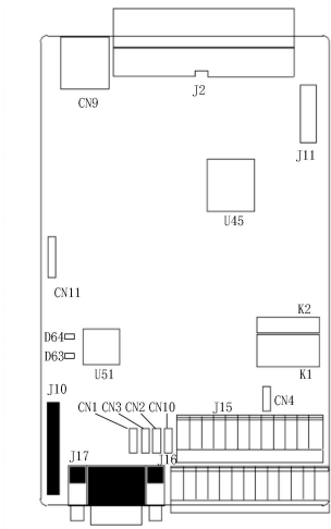
图3-5. 主控板正视图的接线端子及接插件布局图
