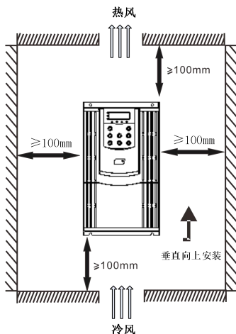
图3-1. 单体安装图
