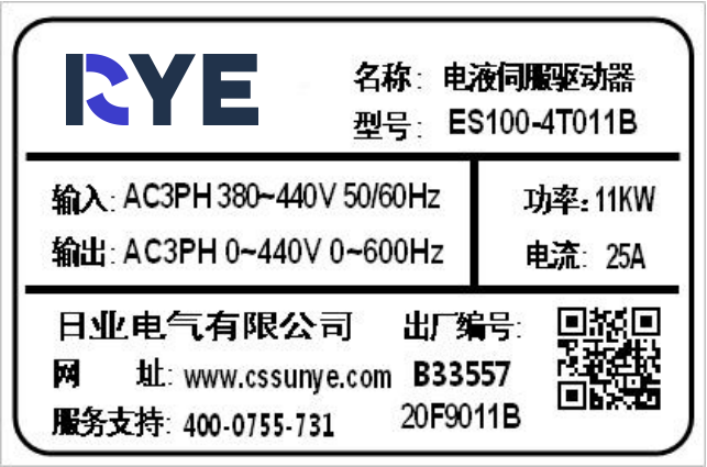
图2-2. 铭牌
