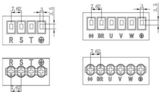
输入端子
