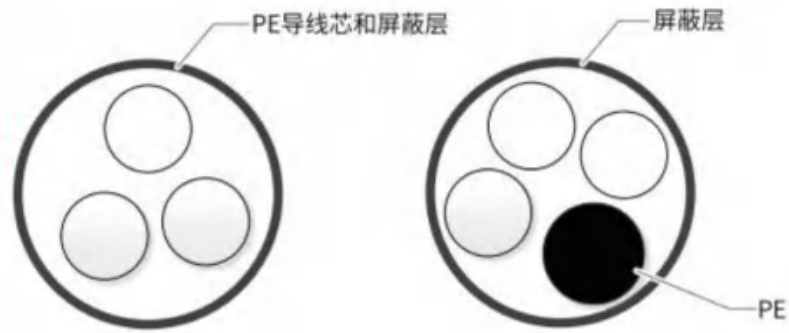
图 4-3 推荐的动力线缆类型
