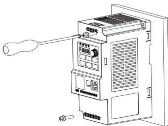
图 5-9 壁挂式安装
