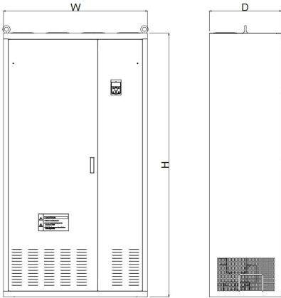
图 2-12. 380V (4T) 500~1000kW 变频器外型尺寸及安装尺寸示意图 660V (7T) 280~710kW 变频器外型尺寸及安装尺寸示意图
