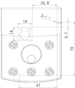
图2-15. 外引键盘不带托盘安装尺寸图
