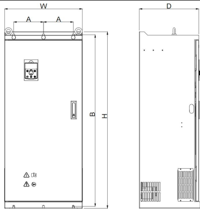
图 2-11. 660V (7T) 75~250kW 变频器外型尺寸及安装尺寸示意图
