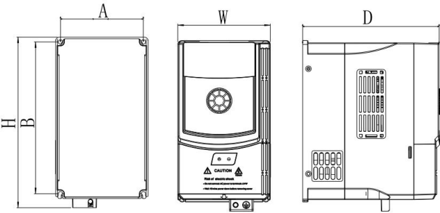
图 2-3. 220V（3S）2.2kW 以下塑胶外形尺寸及安装尺寸示意图 380V（4T）15kW 以下塑胶外形尺寸及安装尺寸示意图
