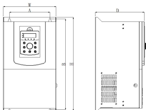
图 2-6. 380V (4T) 18~37kW 钣金机箱外形尺寸及安装尺寸示意图
