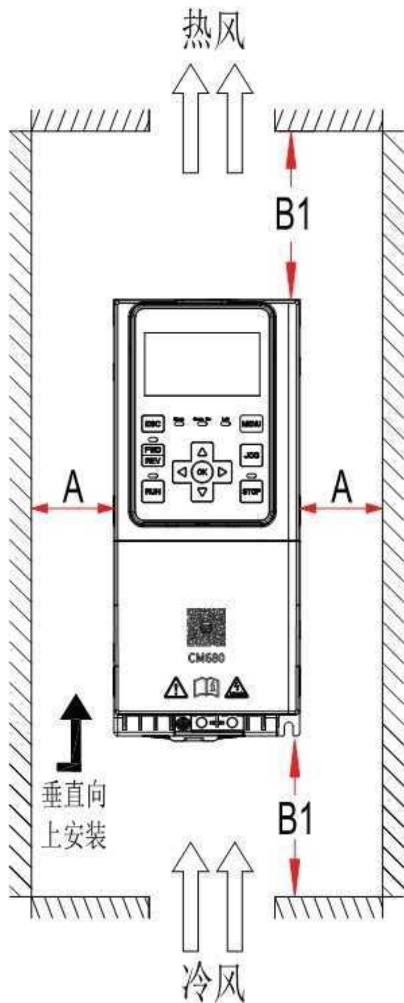
C2~C8机型壁挂安装示意图
