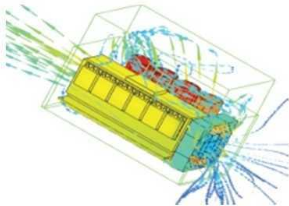
独立风道设计
