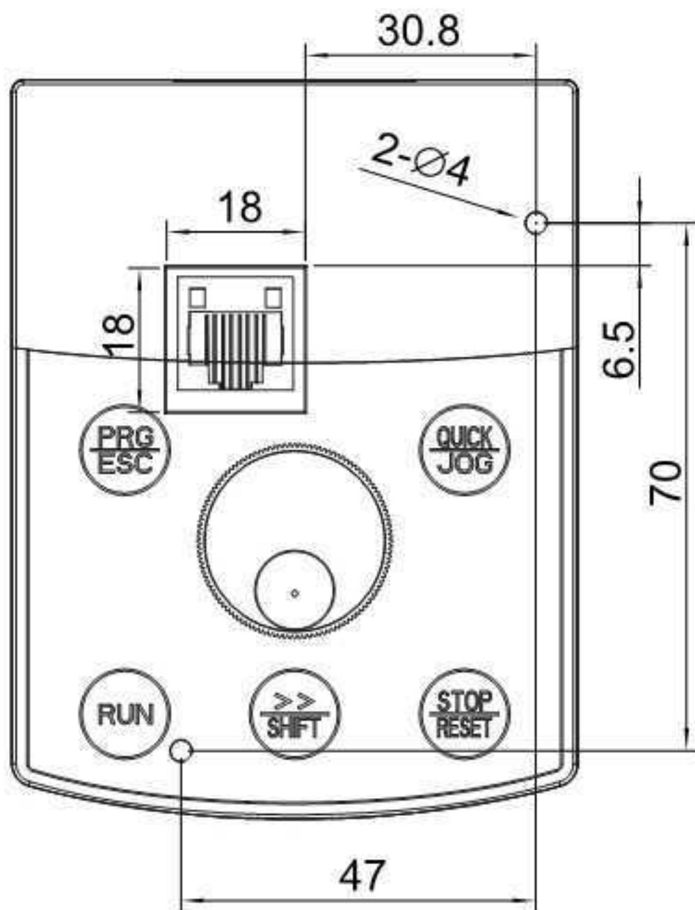
外引键盘不带托盘安装尺寸图
