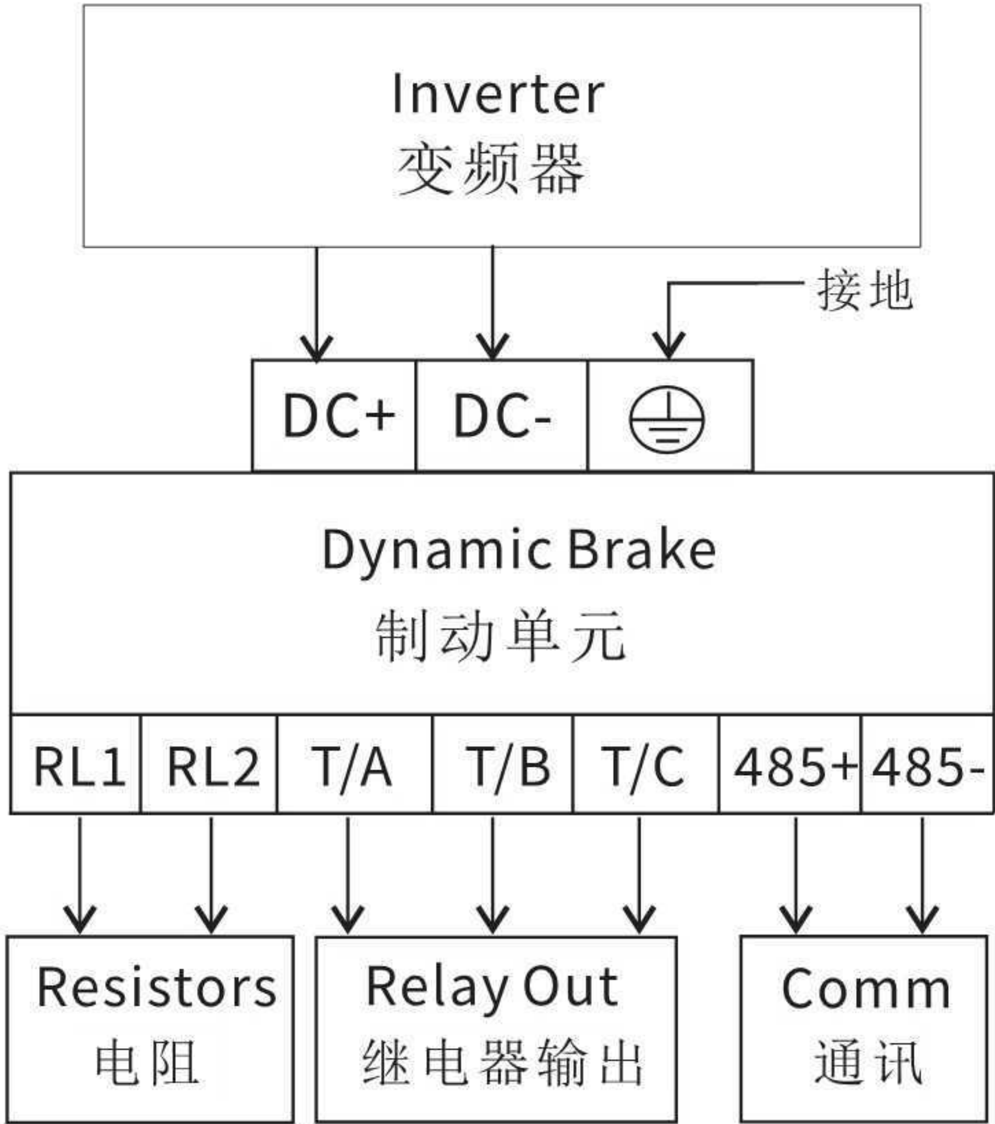
BR530E-4T200以上制动单元接线示意图
