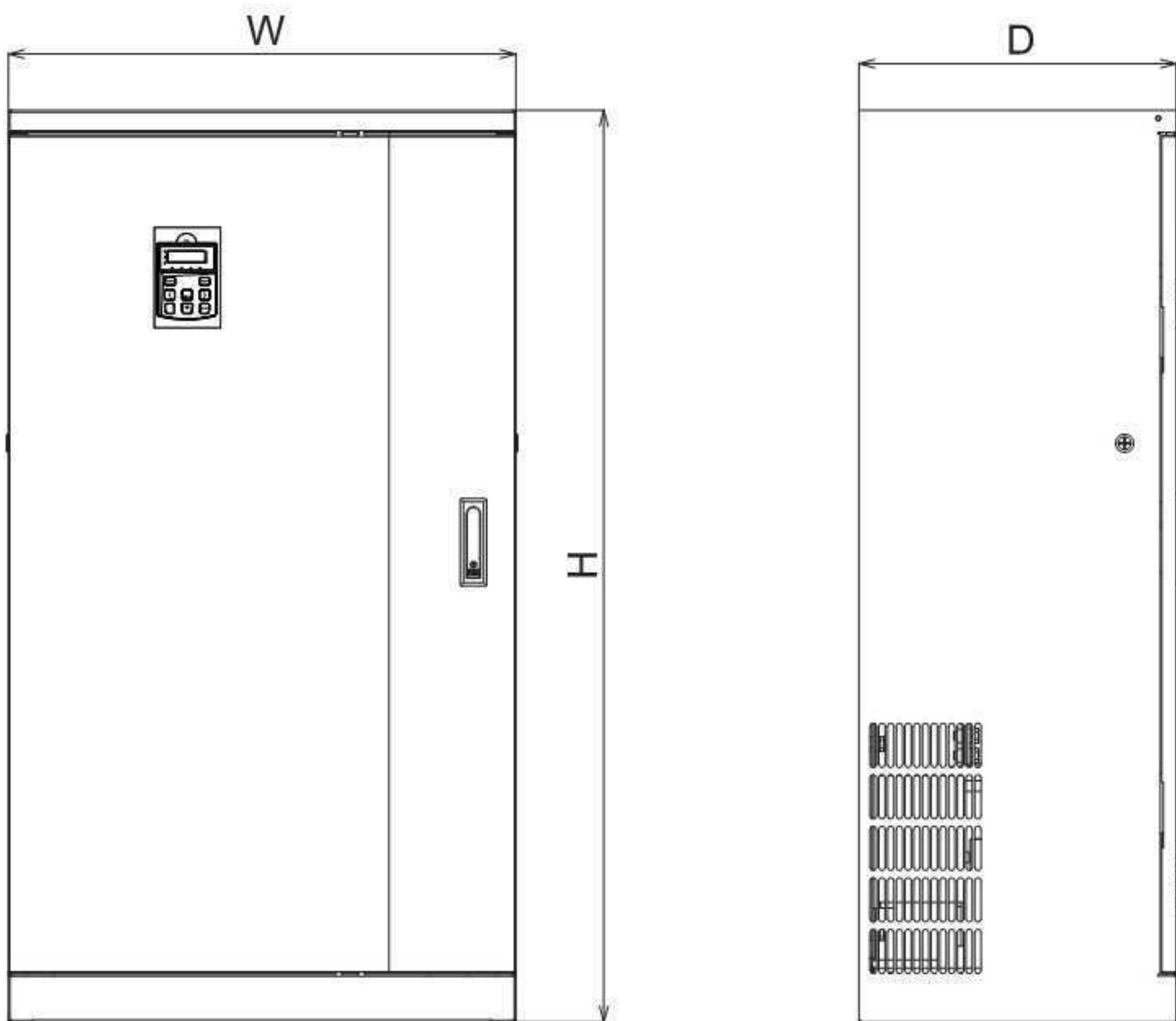
18 ~ 37KW塑壳机箱外形尺寸及安装尺寸示意图
