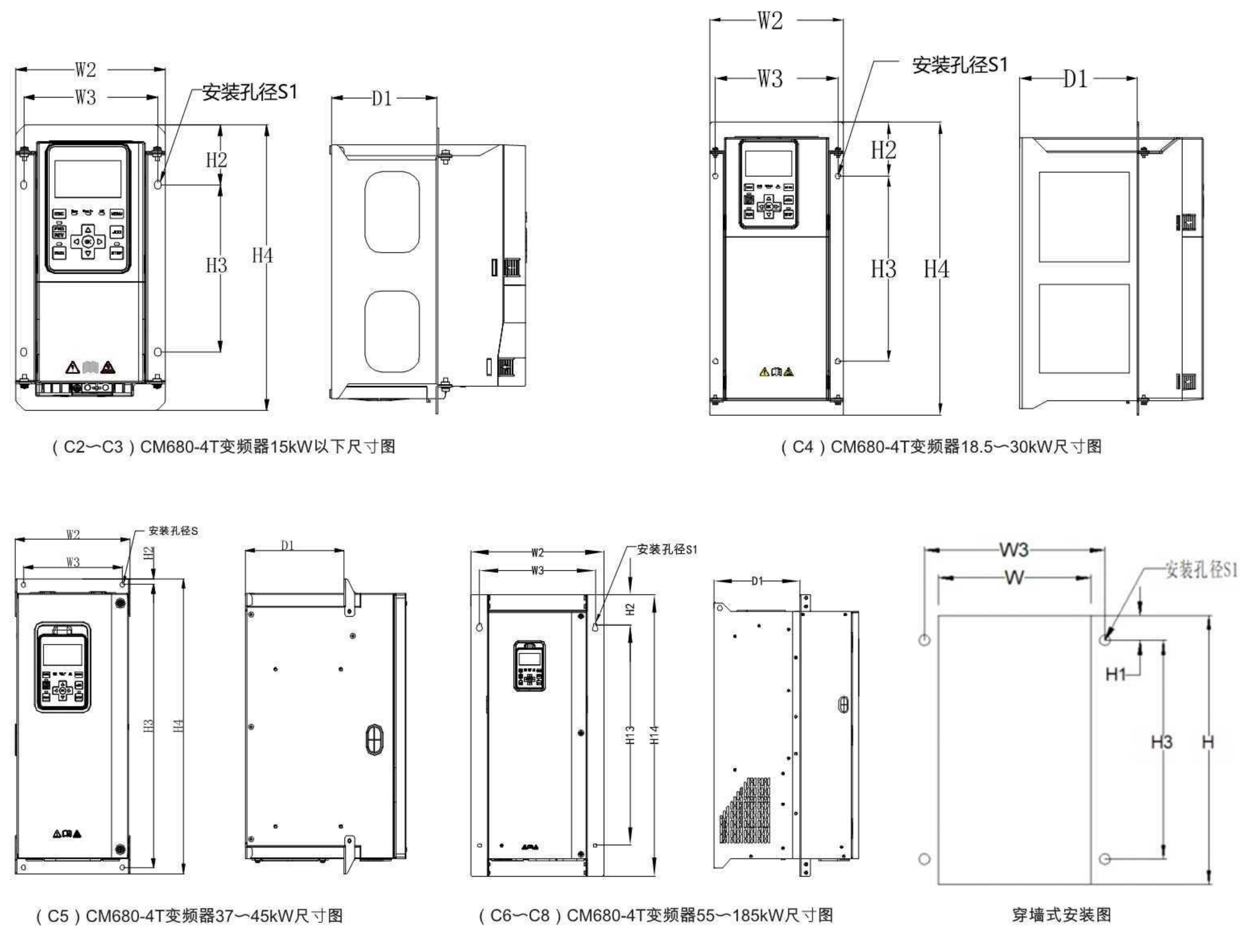
C2-C8穿墙安装尺寸
