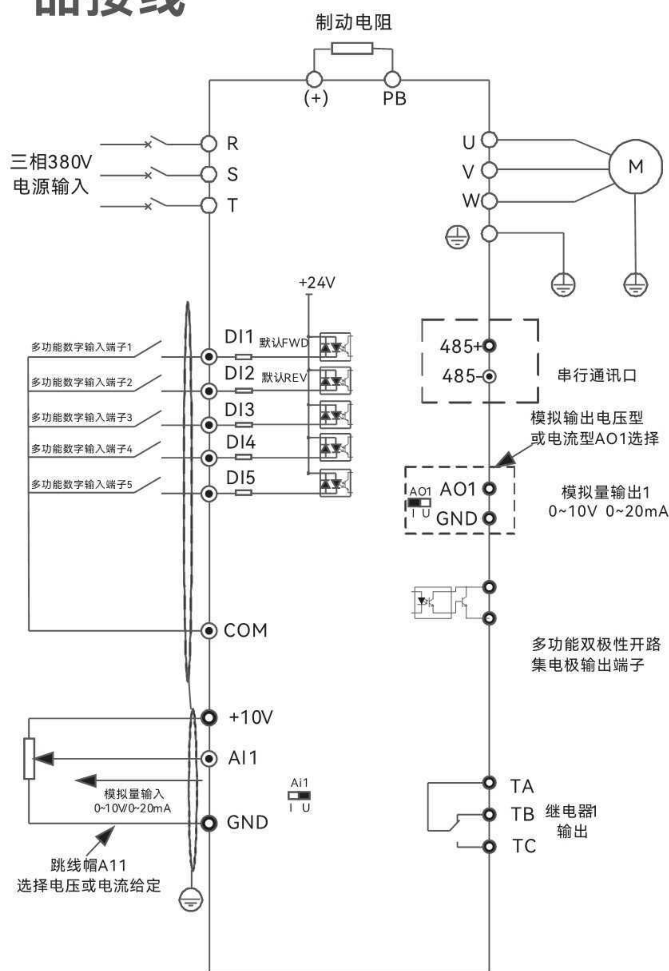
图1.三相（380V）变频器 \leq 9.0\text{kW}
