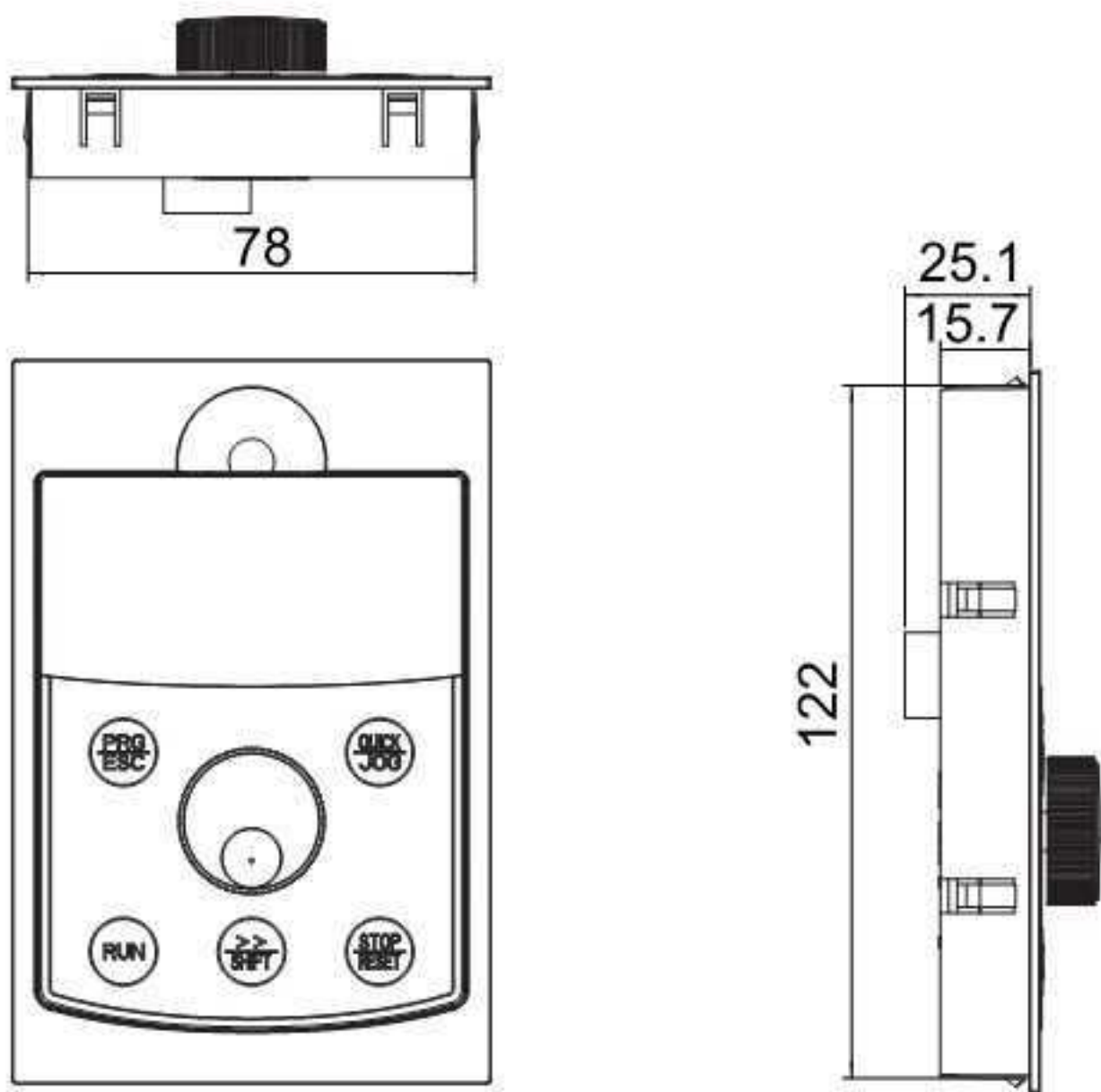
外引键盘带托盘安装尺寸图
