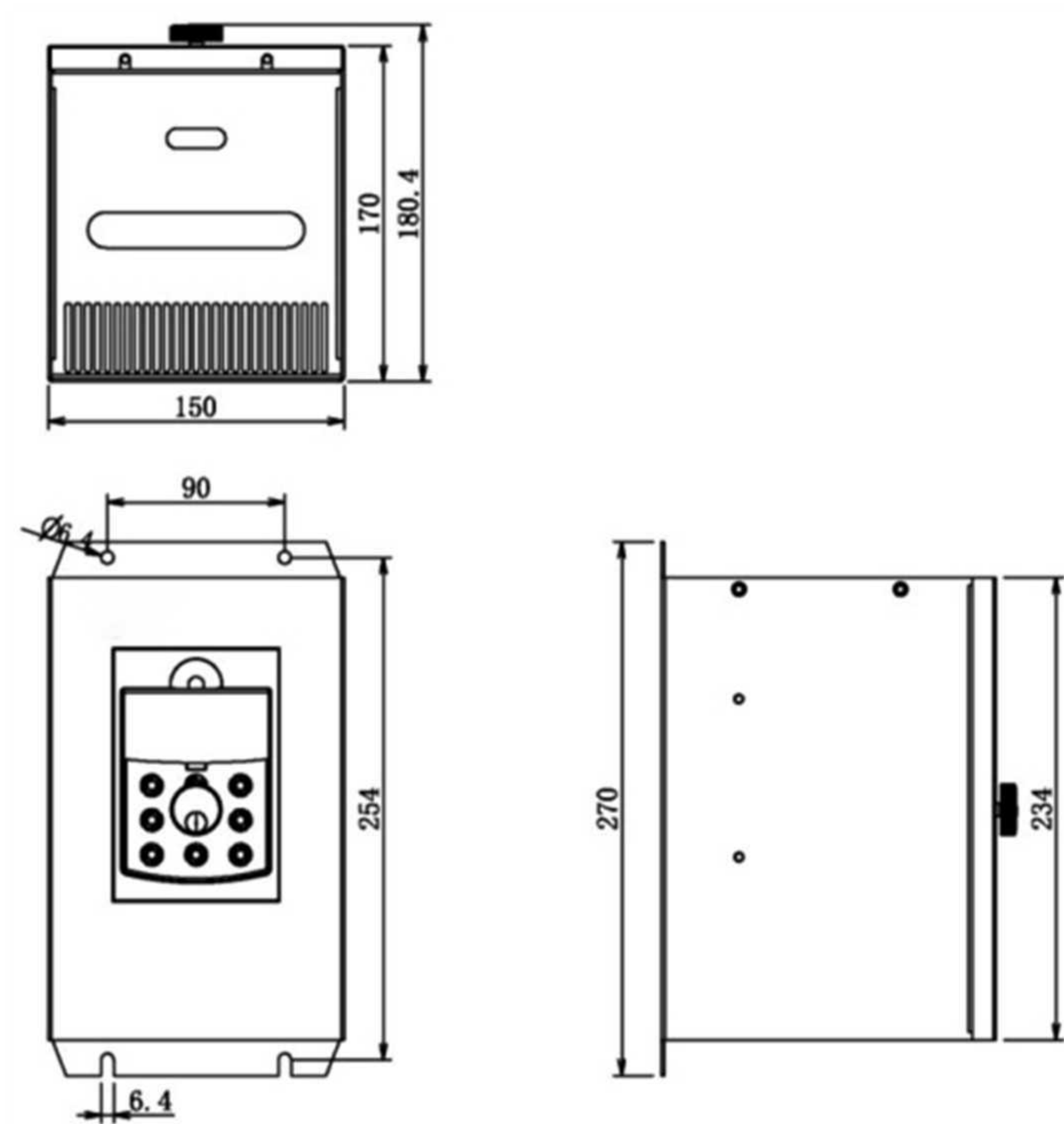
75 ~ 132kW 制动单元
