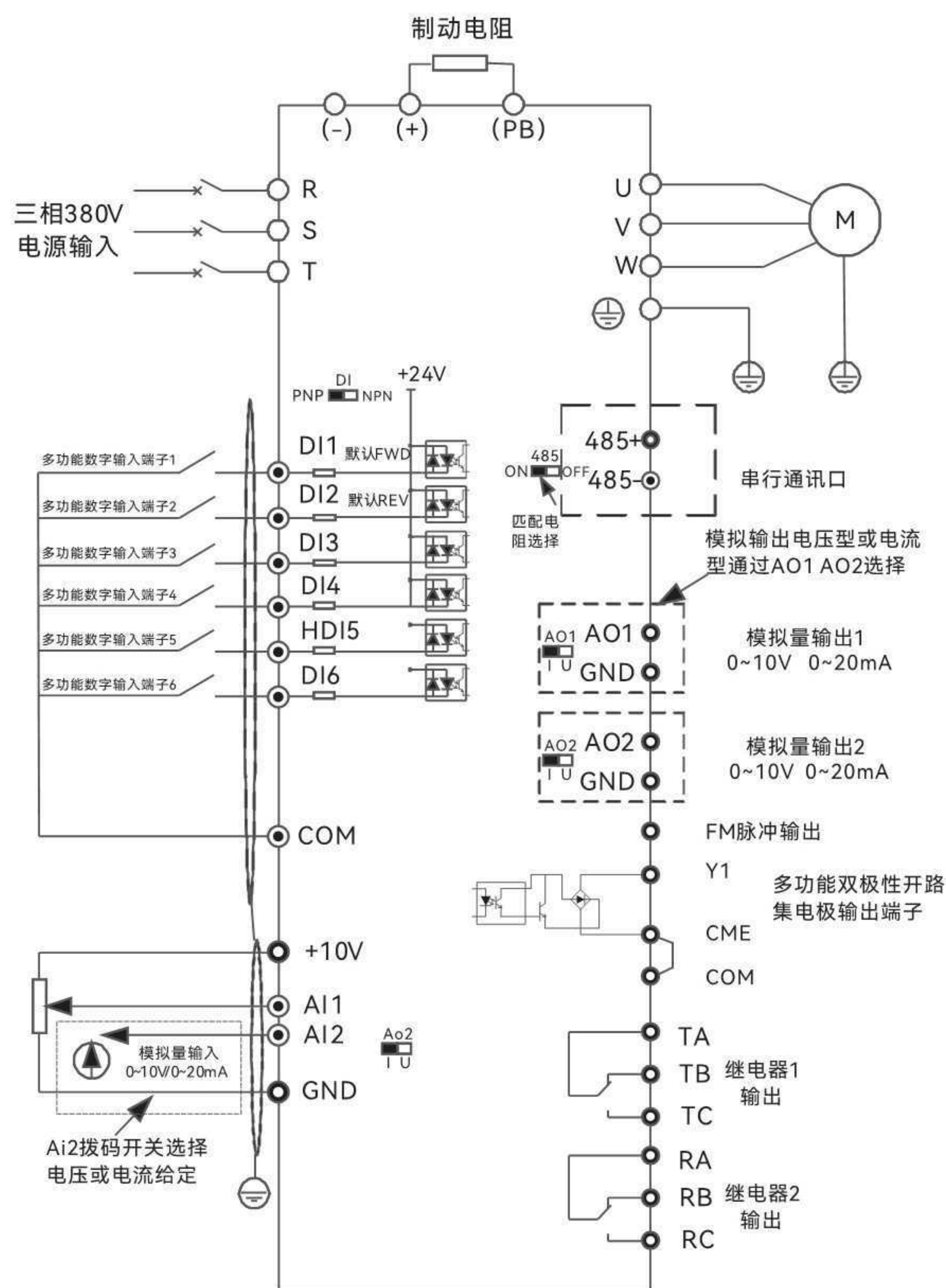
图2. 三相变频器（380V）11kW及以上
