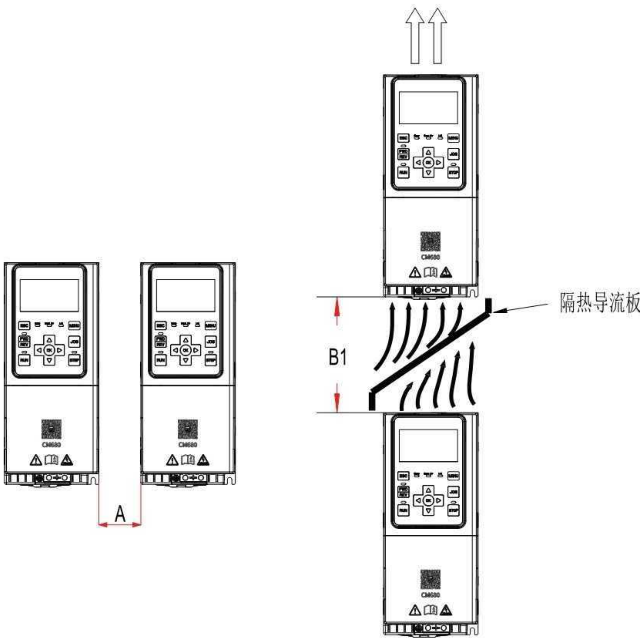
C2~C8机型上下排壁挂安装示意图
