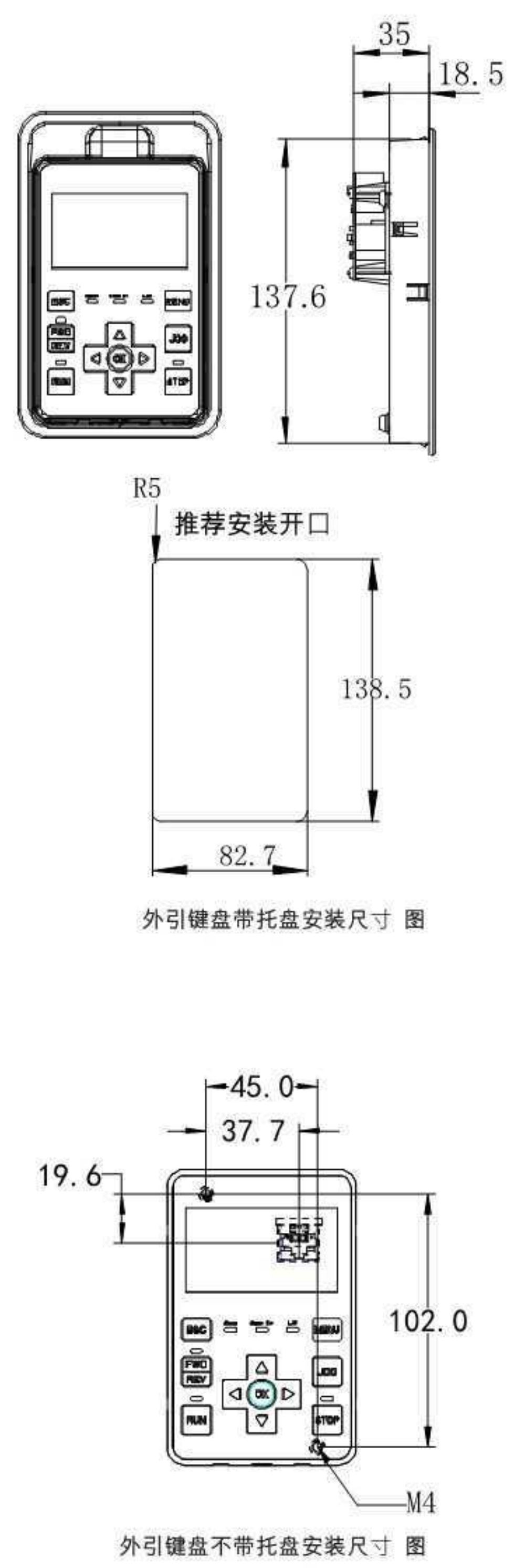
外引键盘安装尺寸图
