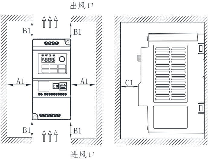
图 5-4 C0~C2 机型安装图（单设备安装）
