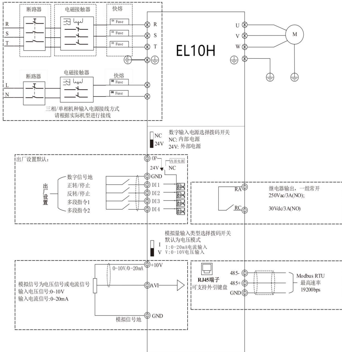
图 6-1 三相/单相电源输入端子接线图
