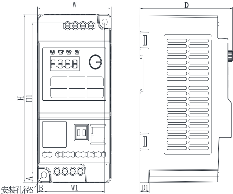
图 5-2 C1 外形及安装尺寸示意图
