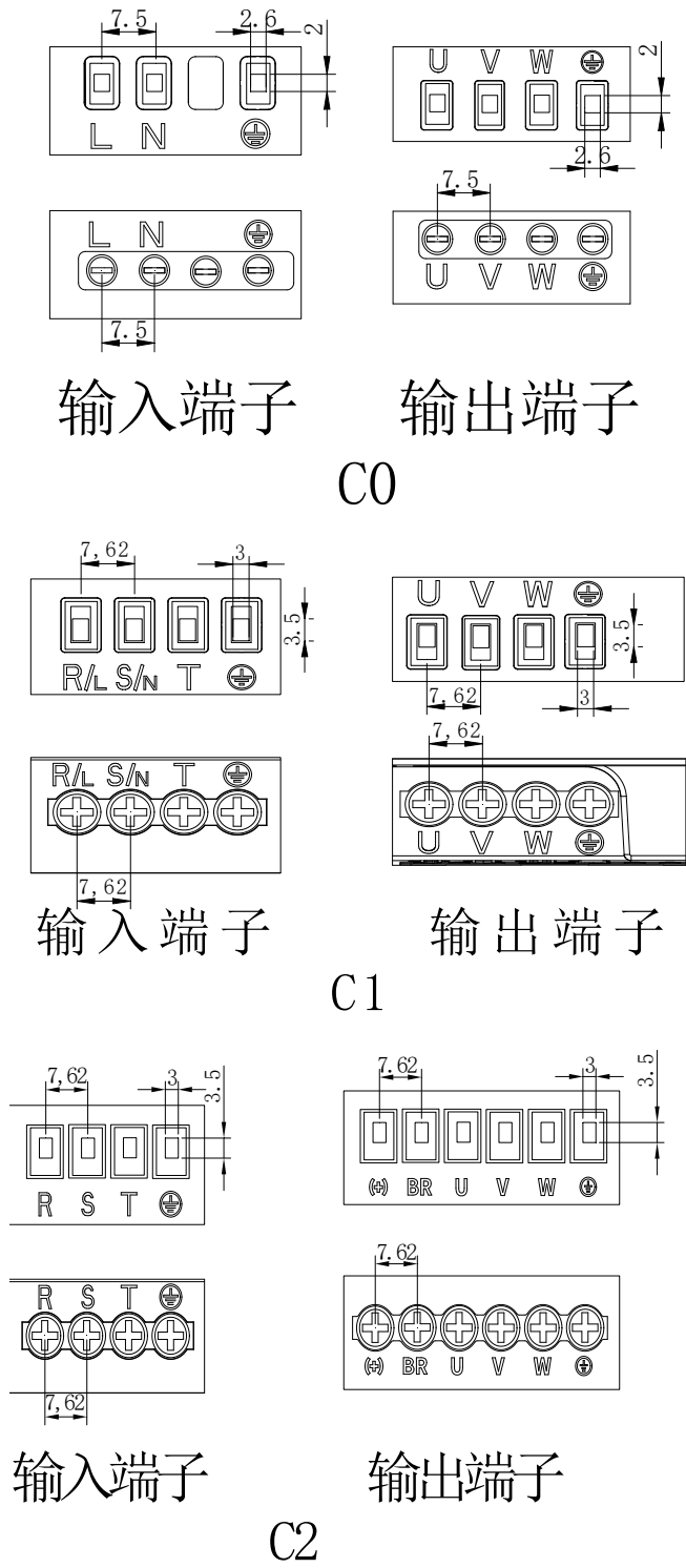
图 6-2 EL10H 变频器主回路端子外形图
