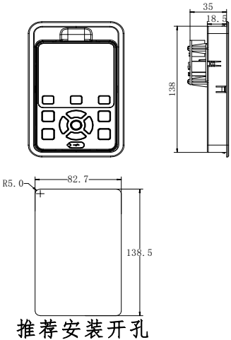
图2-11 外引键盘带托盘安装尺寸图
