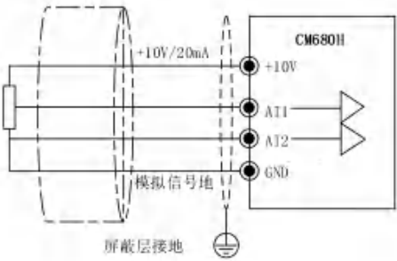
图3-5 模拟量输入端子接线示意图
