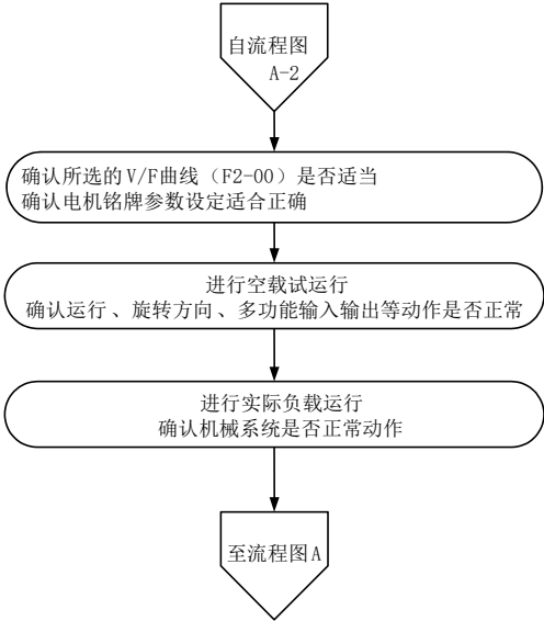
图4-3. V/F控制方式运行步骤
