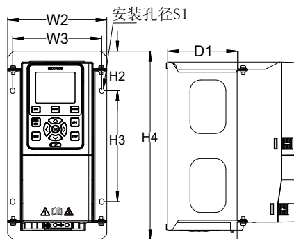
图2-6 (C2 ~ C3) CM680H-4T变频器15kW以下尺寸图
