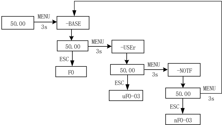
图 5-5. 菜单模式切换操作示意图
