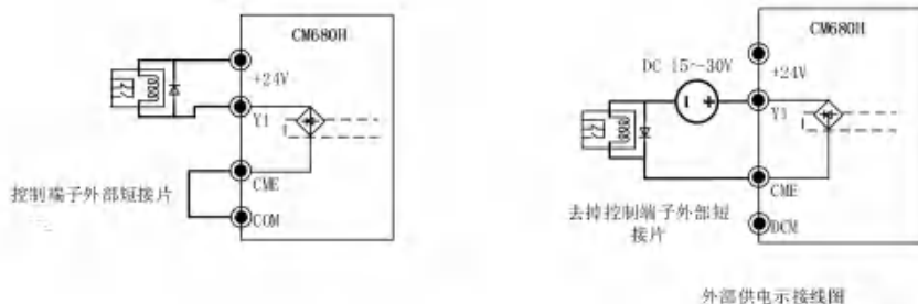
图3-6 数字输出端子Y1接线示意图
