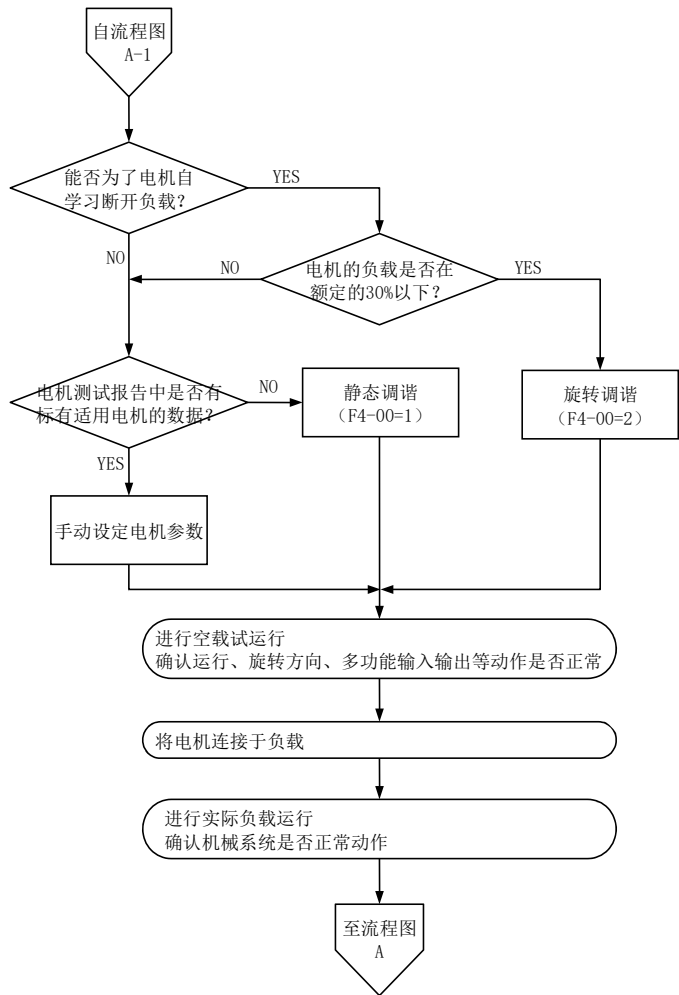
图4-2.闭环矢量控制方式运行步骤
