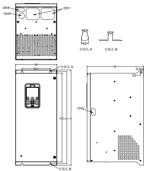
图2-4 (C6~C8) 380V(4T) 55~185kW变频器外型尺寸及安装尺寸示意图
