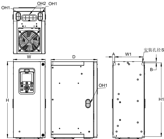
图2-3 (C5) 380V(4T) 37~45kW钣金机箱外形尺寸及安装尺寸示意图
