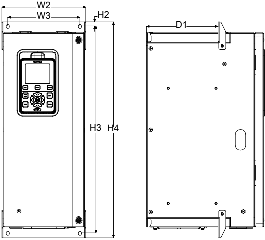
图2-8 (C5) CM680H-4T变频器37~45kW尺寸图
