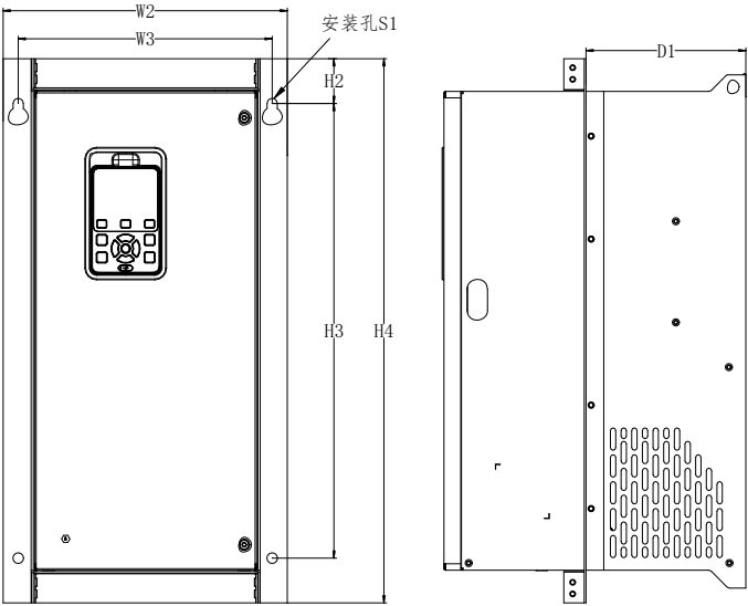
图2-9 (C6~C8) CM680H-4T变频器55~185kW尺寸图
