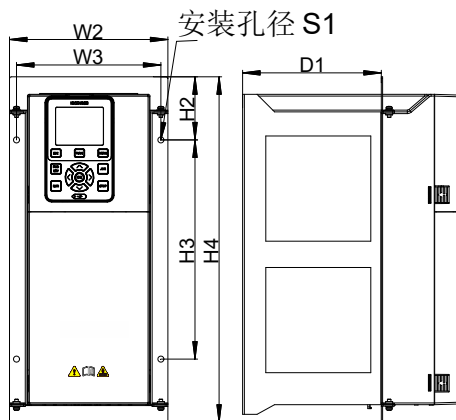
图2-7 (C4) CM680H-4T变频器18.5 ~ 30kW尺寸图
