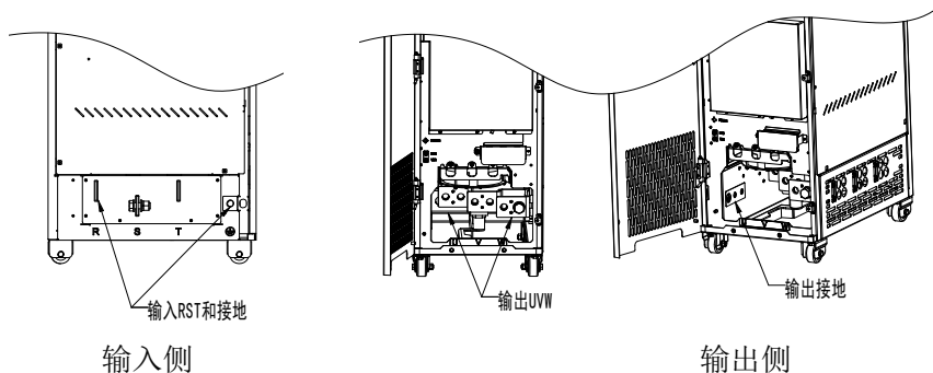
图2-25 变频器接功率线图
