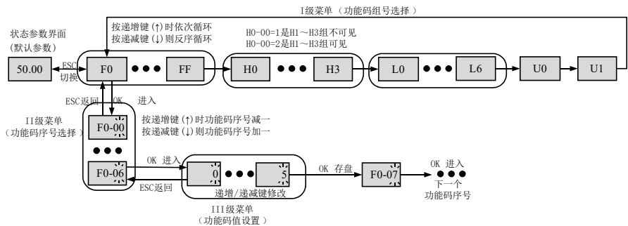
图 5-3. 三级菜单操作流程图
