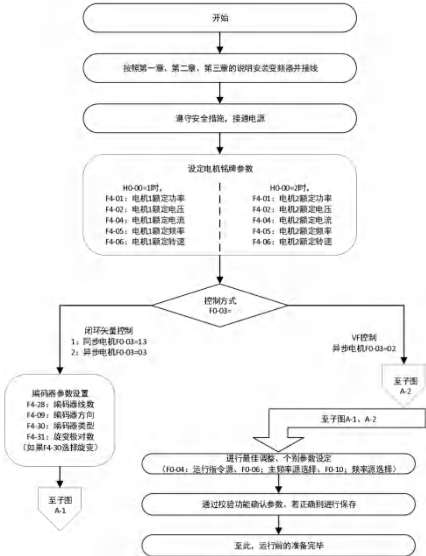
图4-1. 运行前的基本步骤
