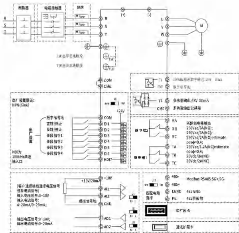
图3-3 160kW~450kW三相变频器
