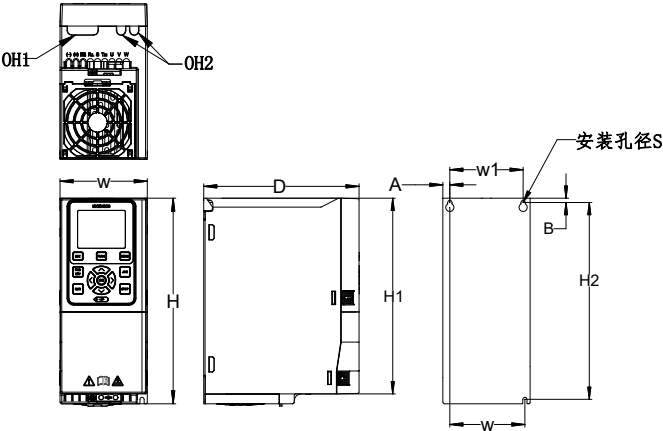
图2-1 (C2 ~ C3) 380V(4T) 15kW以下塑胶外形尺寸及安装尺寸示意图
