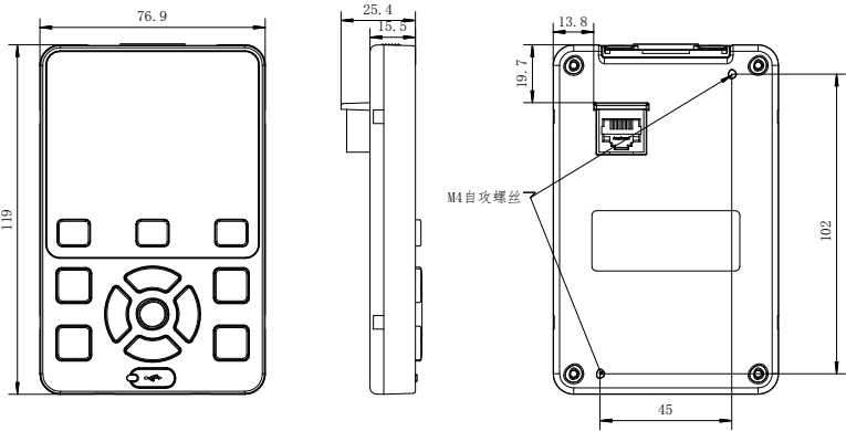
图2-12 外引键盘不带托盘安装尺寸图
