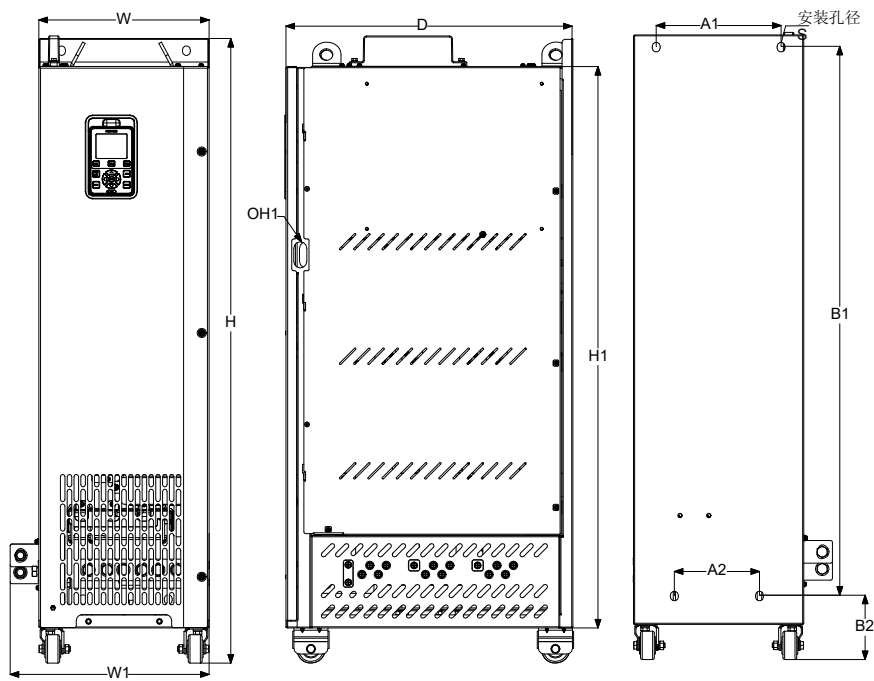
图2-5 (C9~C11) 380V(4T) 200~450kW变频器外形尺寸及安装尺寸示意图
