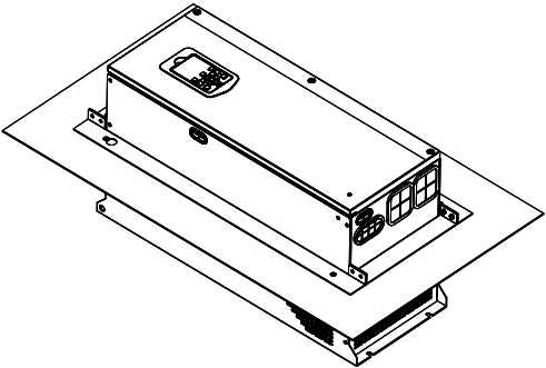
图2-16 钣金结构穿墙式安装方式
