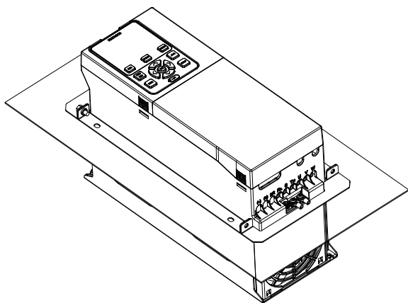
图2-14 塑壳结构穿墙式安装方式
