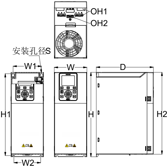
图2-2 (C4) 380V(4T) 18.5 ~ 30kW以下塑胶外形尺寸及安装尺寸示意图
