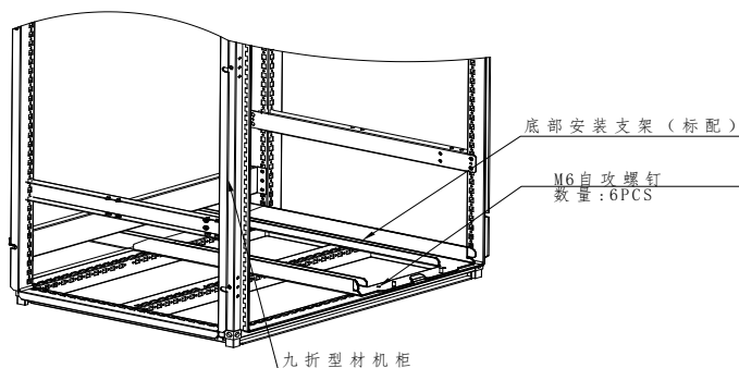
图2-22 底部安装支架安装示意图
