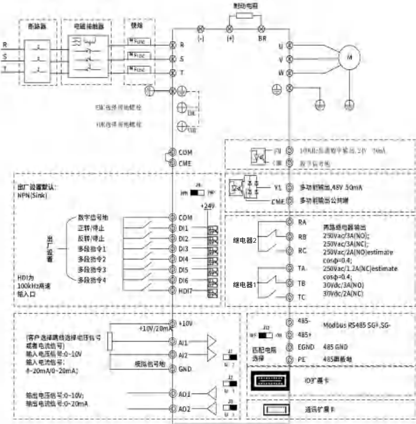
图3-2 11kW ~ 132kW三相变频器
