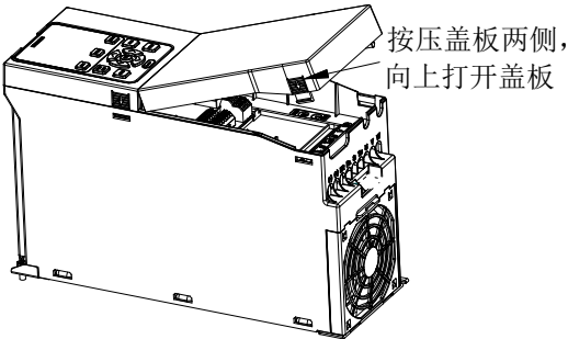
图2-17 塑壳结构端子拆装图
