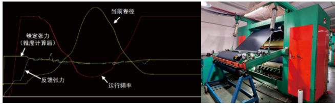
根据线速度等计算卷径,经过锥度计算后 张力给定值随卷径自动调整避免材料发生皱褶或变形
