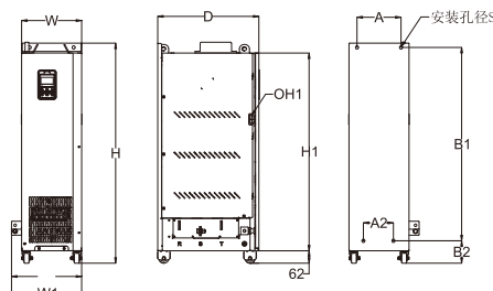
C9~C11) 380V(4T) 200~450kW变频器外形尺寸及安装尺寸示意图
