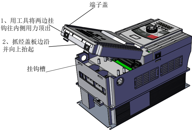
图3-3. 塑胶外壳端子盖拆卸图
