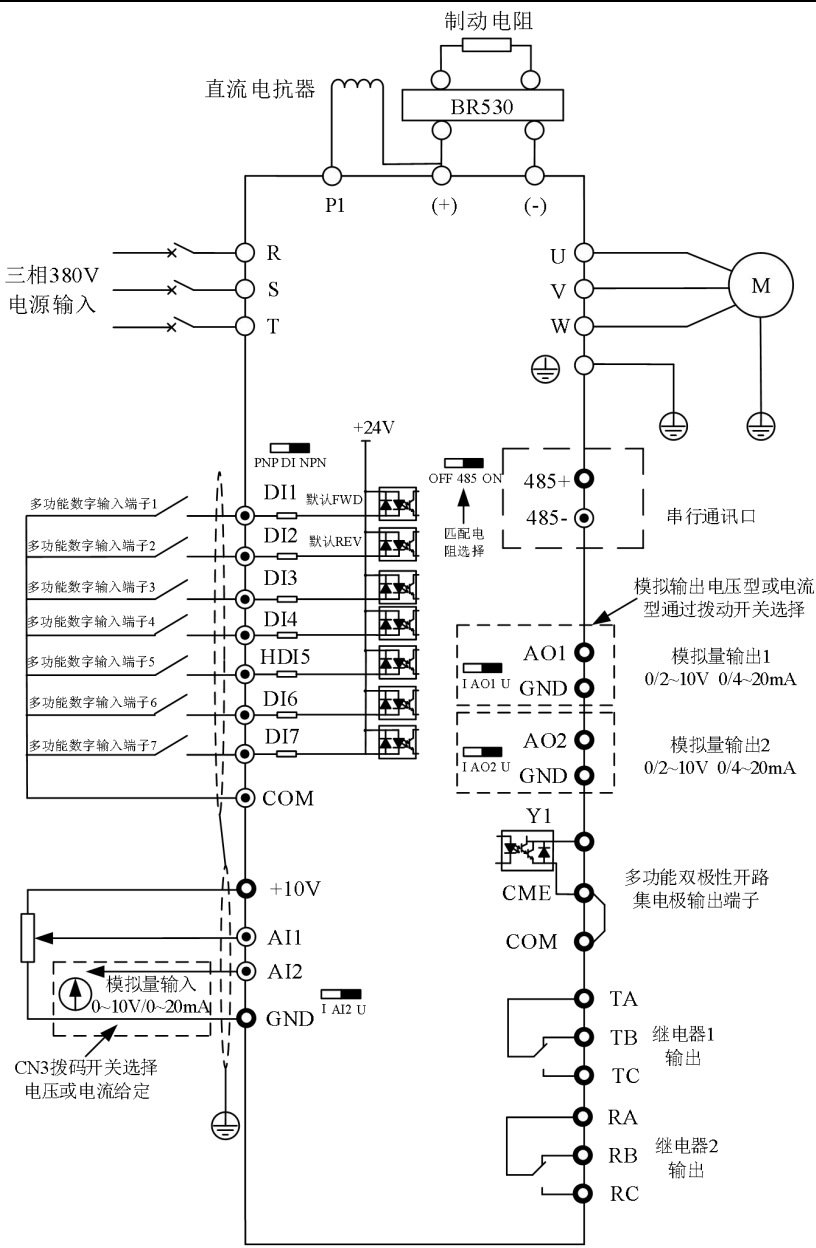
图 3-7. (4T) 75kW 及以上三相变频器
