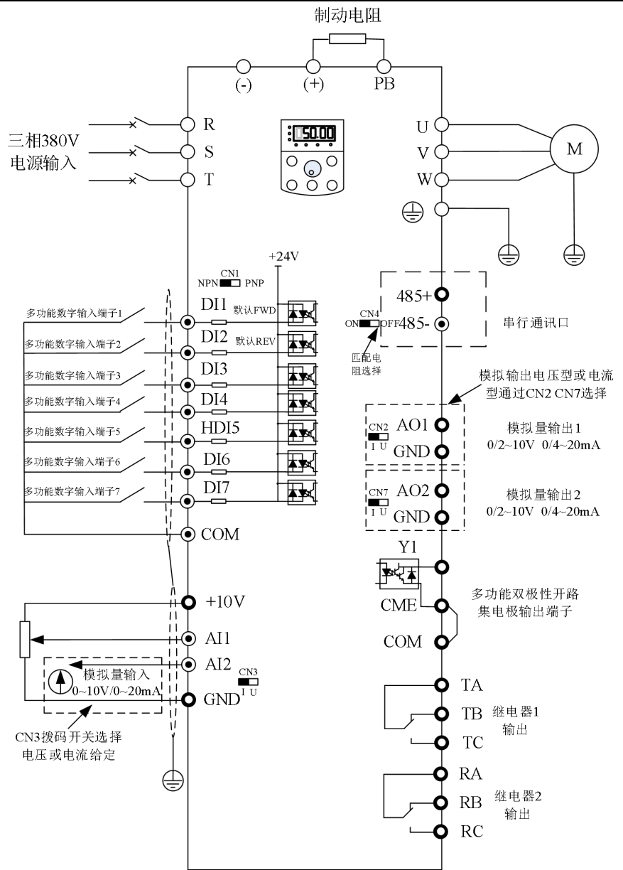
图 3-5. (4T) 4.0~30kW 以下三相变频器
