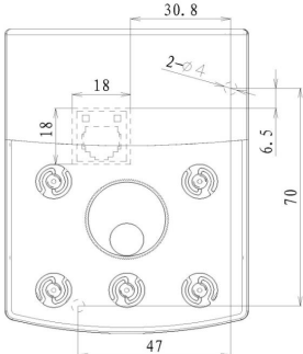
图2-8. 外引键盘不带托盘安装尺寸图
