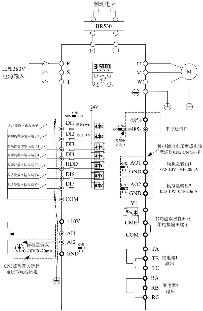
图 3-6. (4T) 37kW ~ 55kW 三相变频器
