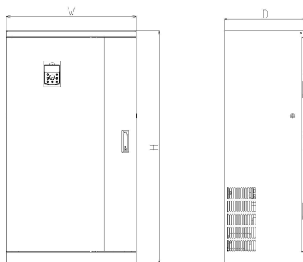
图 2-6. 380V (4T) 355~800kW 变频器外型尺寸及安装尺寸示意图
