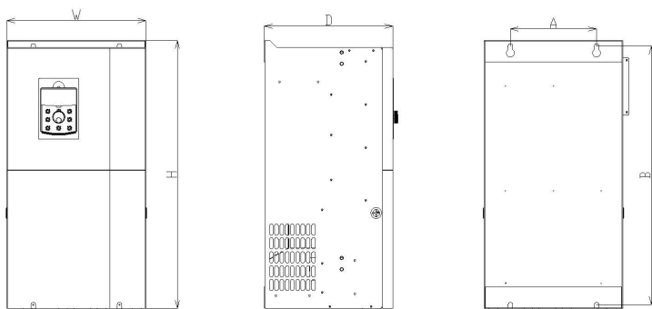
图 2-5. 380V (4T) 45~315kW 变频器外型尺寸及安装尺寸示意图
