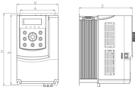
图 2-3. 220V（3S）5.5kW 以下塑胶外形尺寸及安装尺寸示意图 380V（4T）15kW 以下塑胶外形尺寸及安装尺寸示意图
