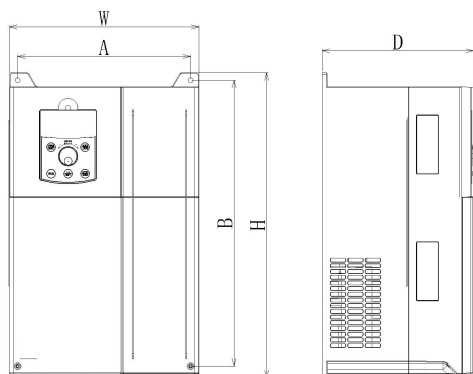
图 2-4. 380V (4T) 18~37kW 塑壳机箱外形尺寸及安装尺寸示意图
