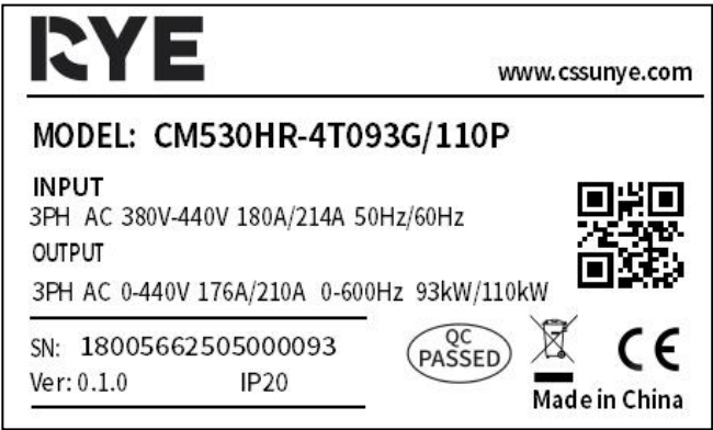
图2-2. 铭牌
