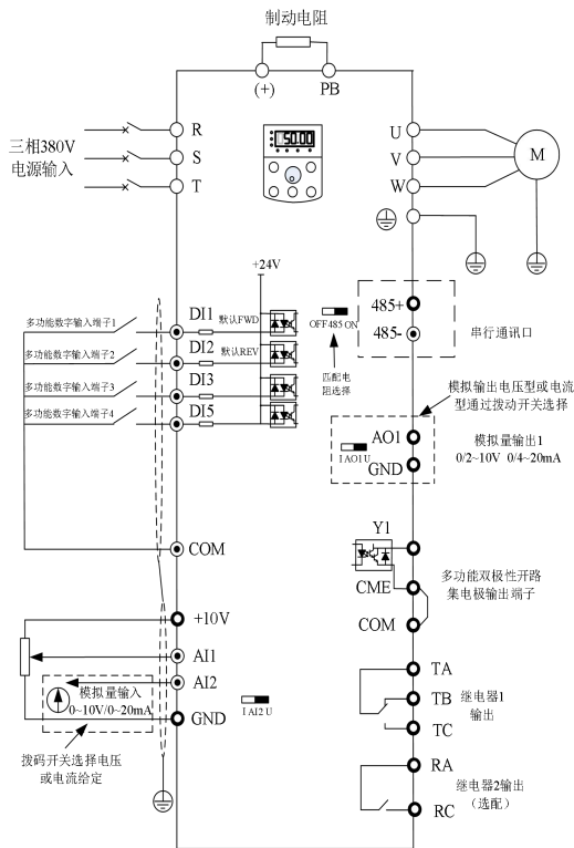
图 3-4. 2.2kW 及其以下三相变频器
