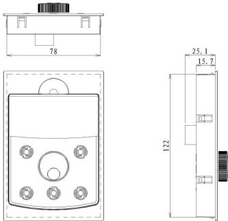
图2-7. 外引键盘带托盘安装尺寸图
