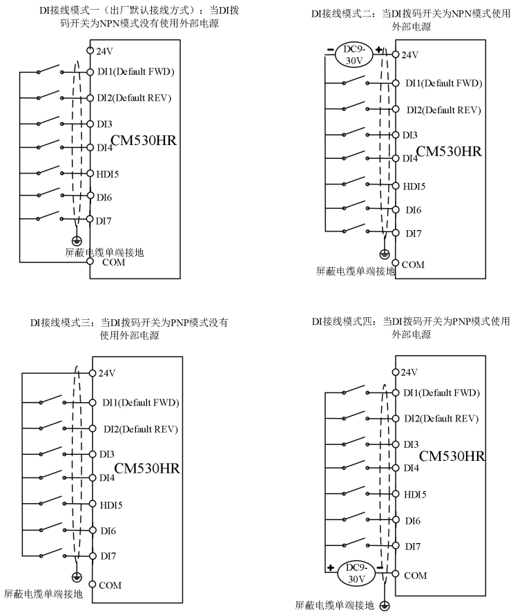
图3-9. 四种不同模式下数字输入端子接线图
