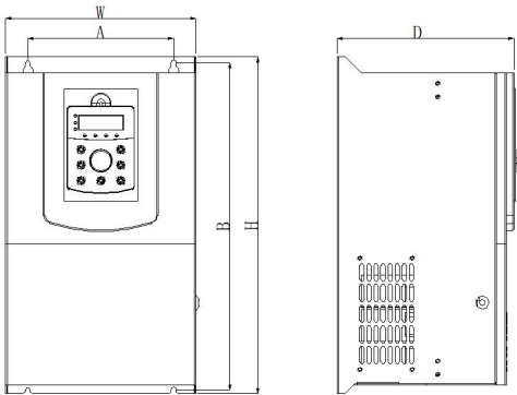
图 2-6. 380V (4T) 18~37kW 钣金机箱外形尺寸及安装尺寸示意图 660V (7T) 11~22kW 钣金机箱外形尺寸及安装尺寸示意图
