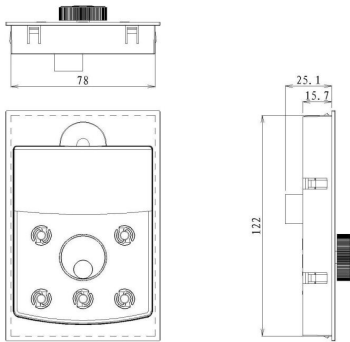
图2-11. 外引键盘带托盘安装尺寸图
