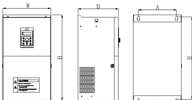
图 2-7. 380V (4T) 45~132kW 变频器外型尺寸及安装尺寸示意图 660V (7T) 30~55kW 变频器外型尺寸及安装尺寸示意图
