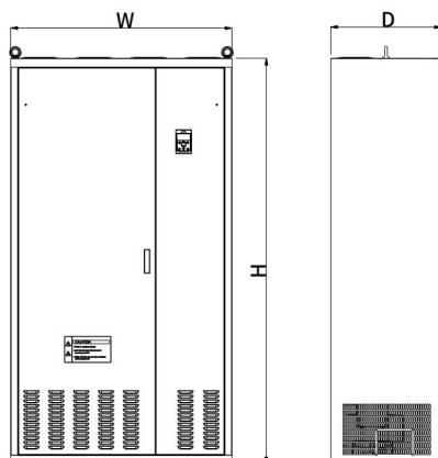
图 2-9. 380V (4T) 500~800kW 变频器外型尺寸及安装尺寸示意图 660V (7T) 500~710kW 变频器外型尺寸及安装尺寸示意图
