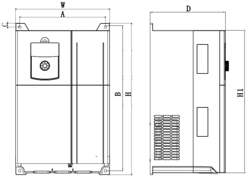
图 2-5. 380V (D4T) 18~37kW 塑壳机箱外形尺寸及安装尺寸示意图
