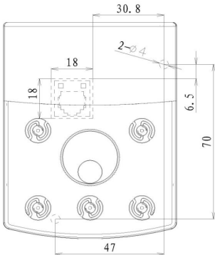
图2-12. 外引键盘不带托盘安装尺寸图
