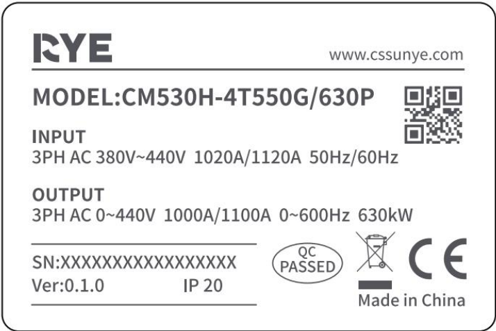
图2-2. 铭牌
