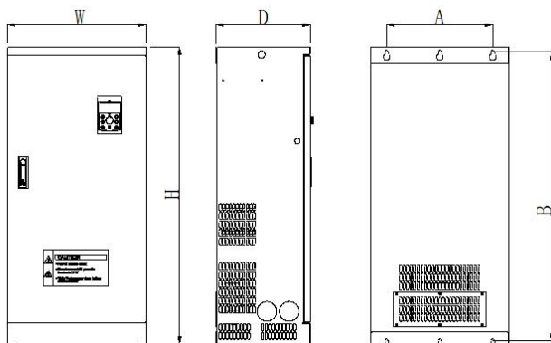
图 2-8. 380V (4T) 160~450kW 变频器外型尺寸及安装尺寸示意图 660V (7T) 75~450kW 变频器外型尺寸及安装尺寸示意图
