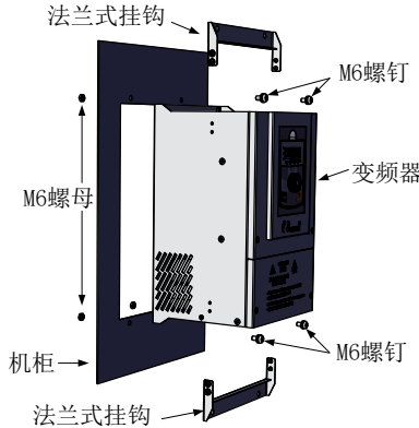
图3-3. CM530H-4T变频器钣金结构45~55kW穿墙式安装图
