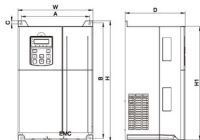
18 ~ 37KW型壳式箱外形尺寸及安装尺寸示意图
