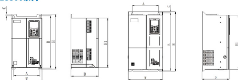
30~37kW钣金机箱外形尺寸及安装尺寸示意图
