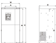
45 ~ 132KW变频器外形尺寸及安装尺寸示意图
