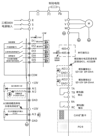
接线方式图
