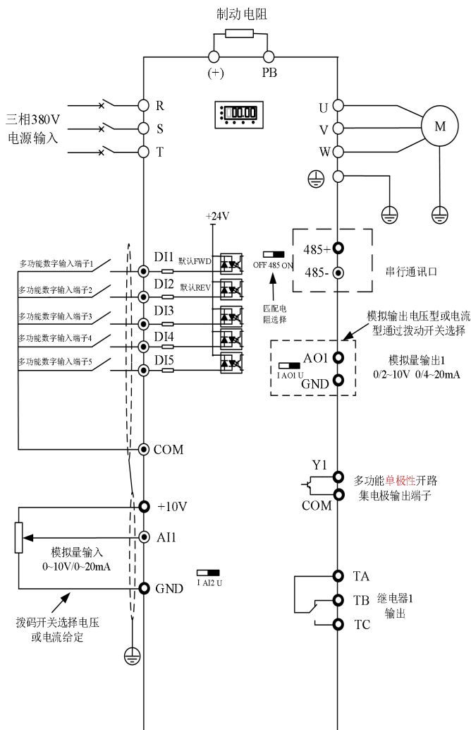
图 3-1. 三相 (380V) 变频器 \leq 9.0\text{kW}
