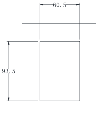
图2-5. 外引键盘带托盘安装开孔尺寸
