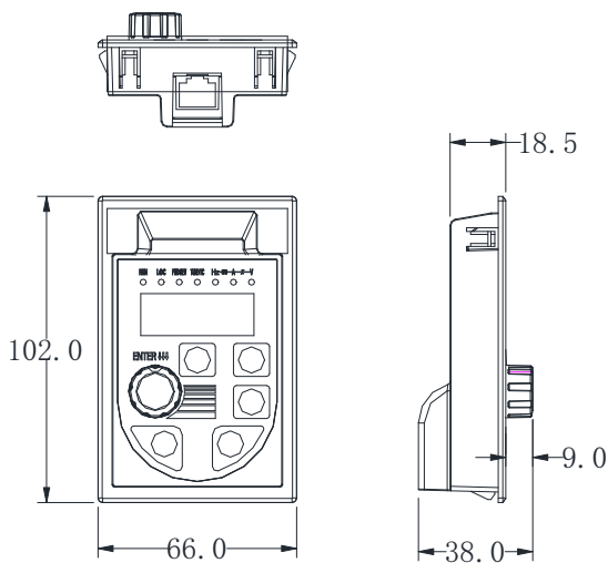
图2-4. 外引键盘带托盘安装尺寸图
