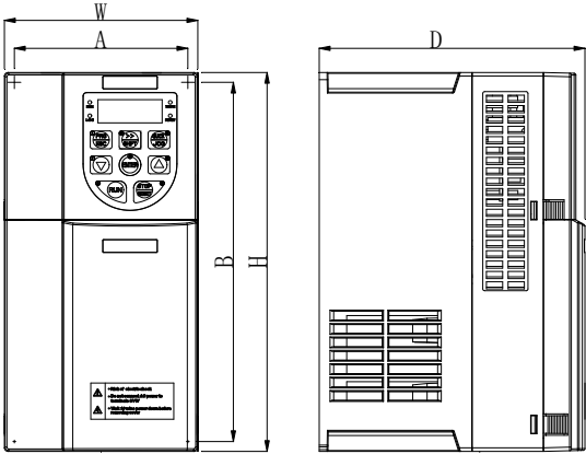
图 2-3. 22KW 以下塑胶外形尺寸及安装尺寸示意图
