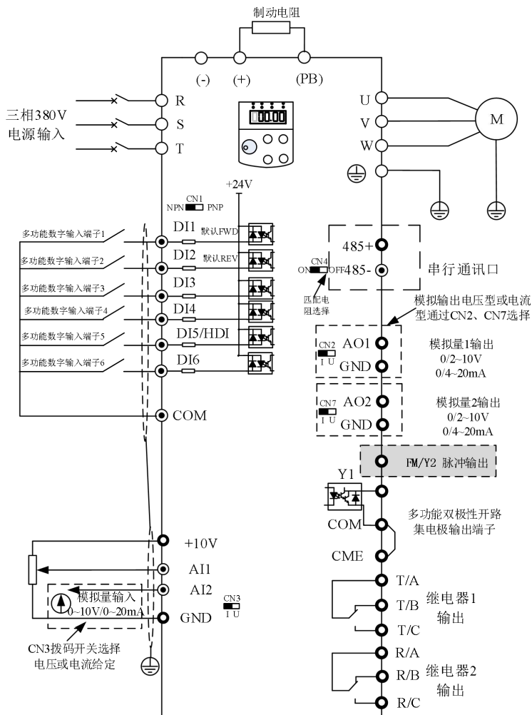
图 3-2. 三相变频器 (380V) \geq 11.0\text{kW}
