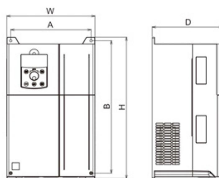
22~37KW钣金机箱外形尺寸及安装尺寸示意图
