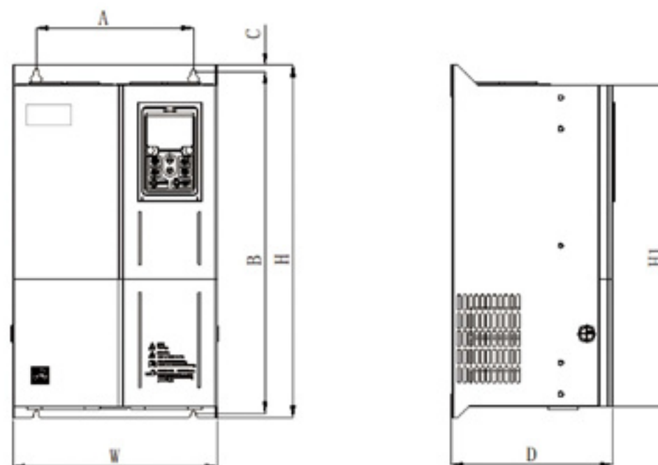
30-37kW钣金机箱外形尺寸及安装尺寸示意图
