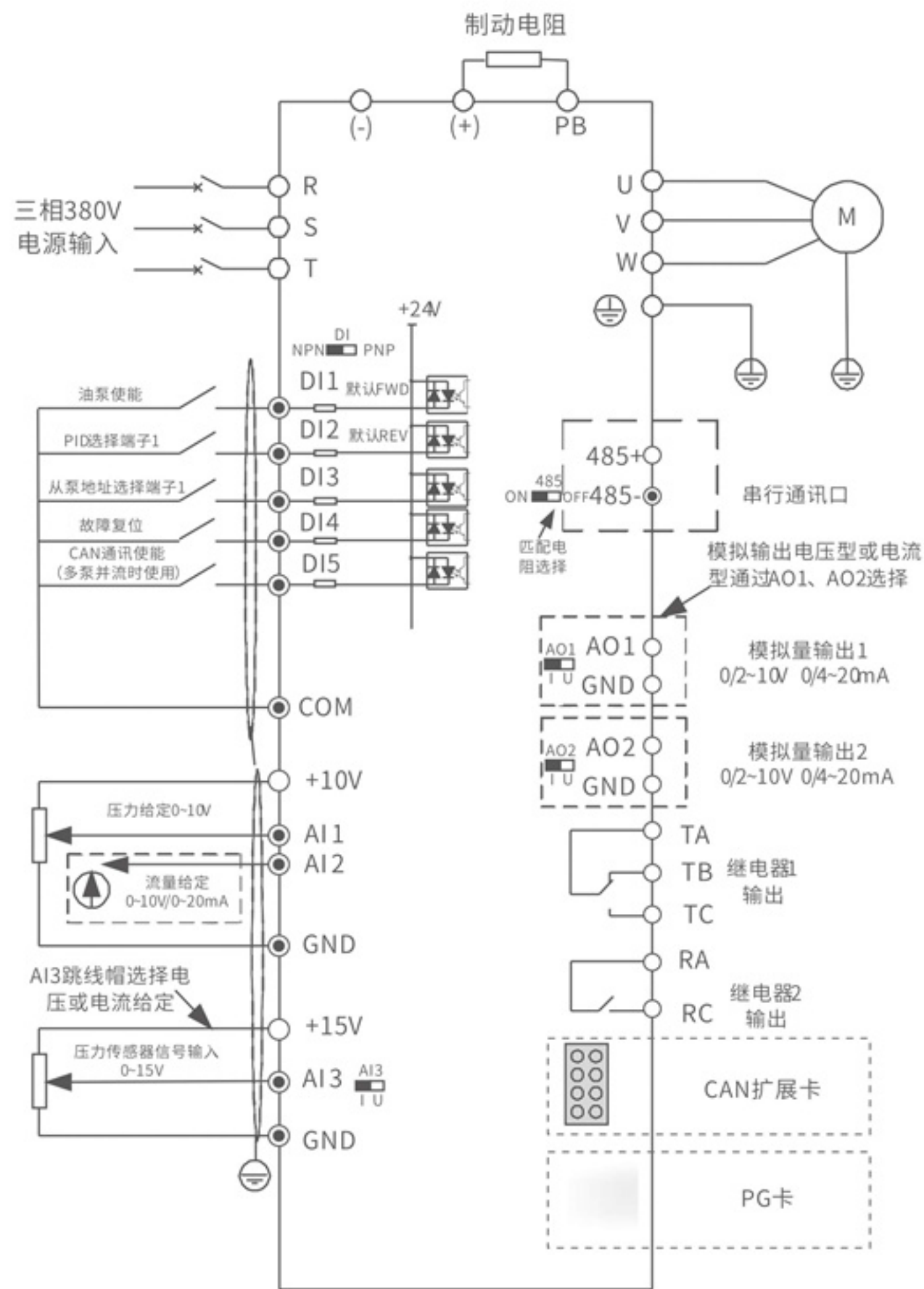
接线方式图
