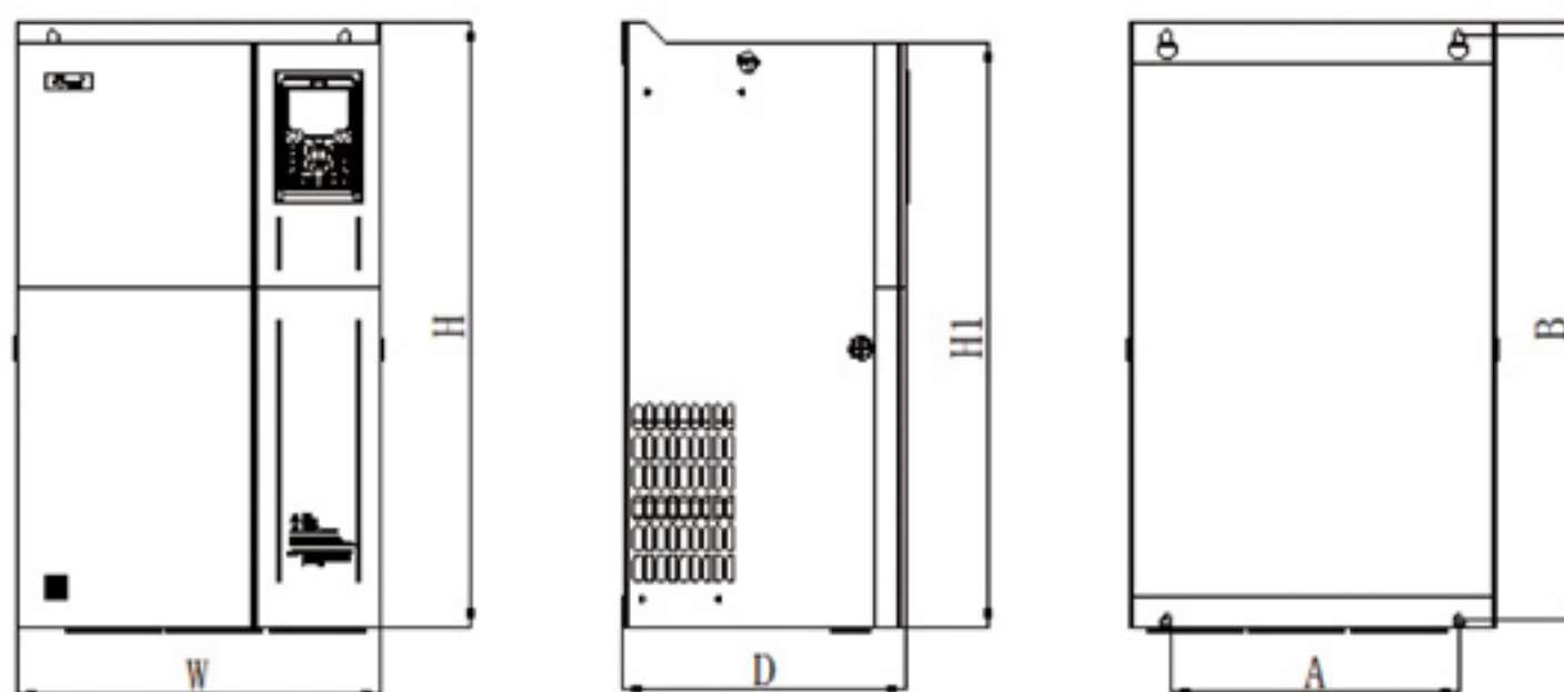
45~132kW变频器外型尺寸及安装尺寸示意图
