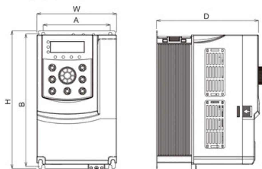
11~18KW塑壳机箱外形尺寸及安装尺寸示意图
