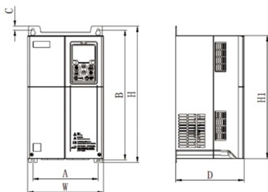
11~22kW塑壳机箱外形尺寸及安装尺寸示意图
