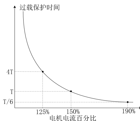
图 10-37 反时限曲线 1
