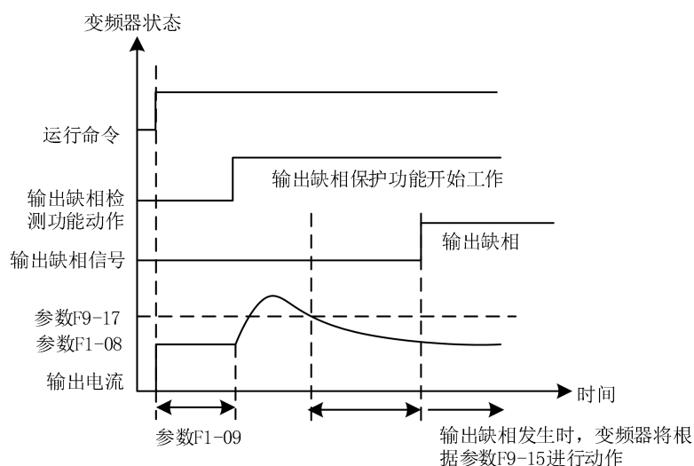
图 9-27 F9-18=0 且 F1-09≠0
