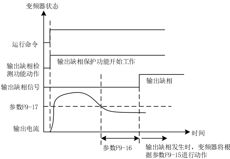
图 10-42 F9-18=0
