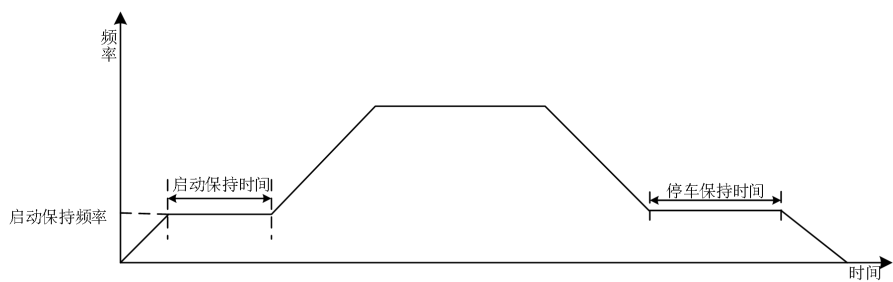
图 10-32 频率保持
