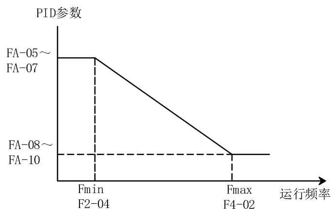
图 9-37 PI 参数调节示意图
