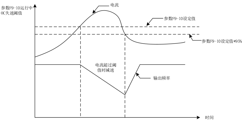
图 10-26 恒速中过流失速
