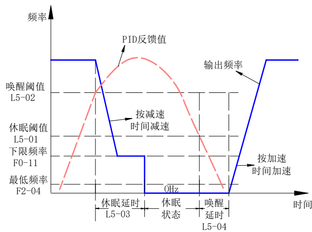
图 10-36 PID 反馈值
