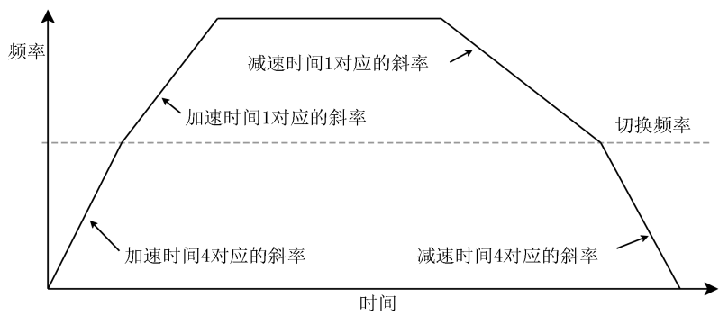
图 9-4 1-4 段加减速频率切换点
