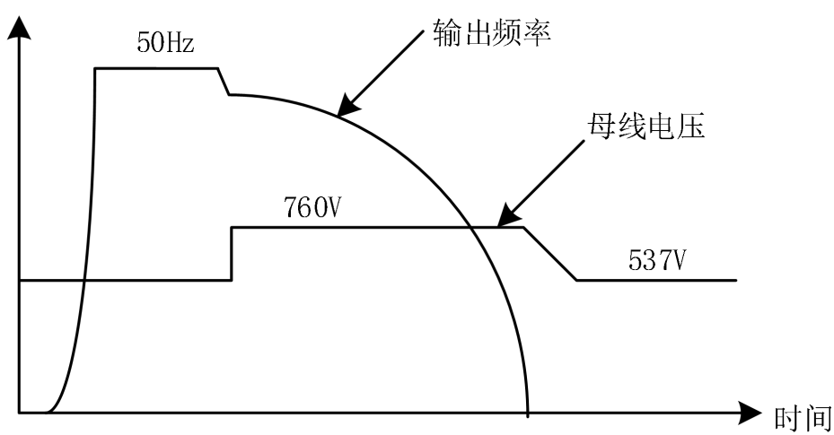
图 10-27 过压失速防止方法 1
