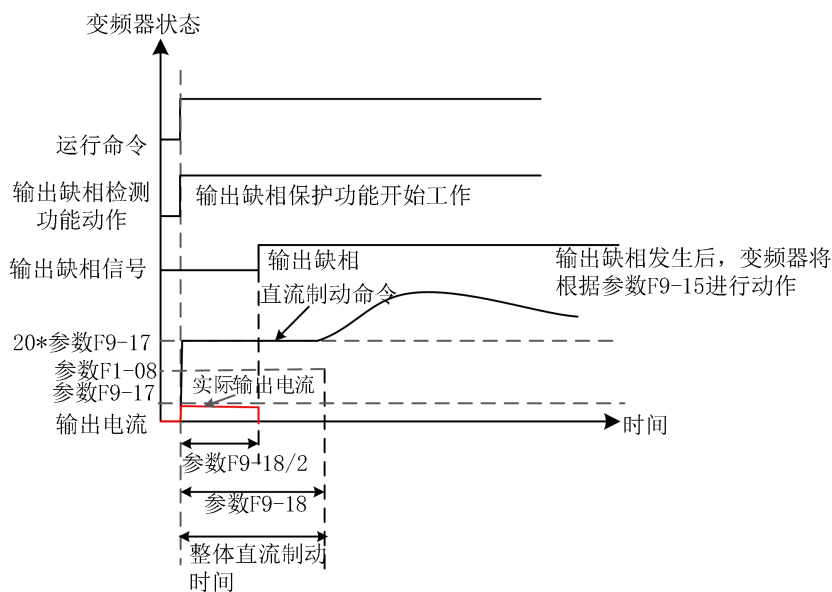
图 10-47 F9-18 \neq 0 且 F1-09=0 (启动时检测到输出缺相)
