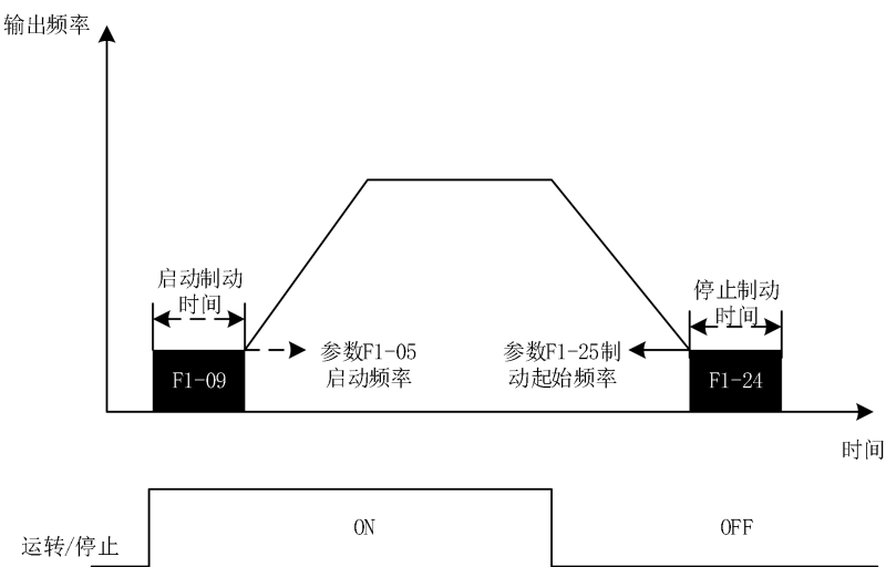
图 9-3 直流/停止制动功能
