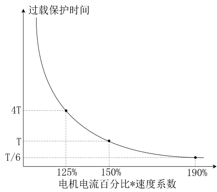
图 10-38 反时限曲线 2
