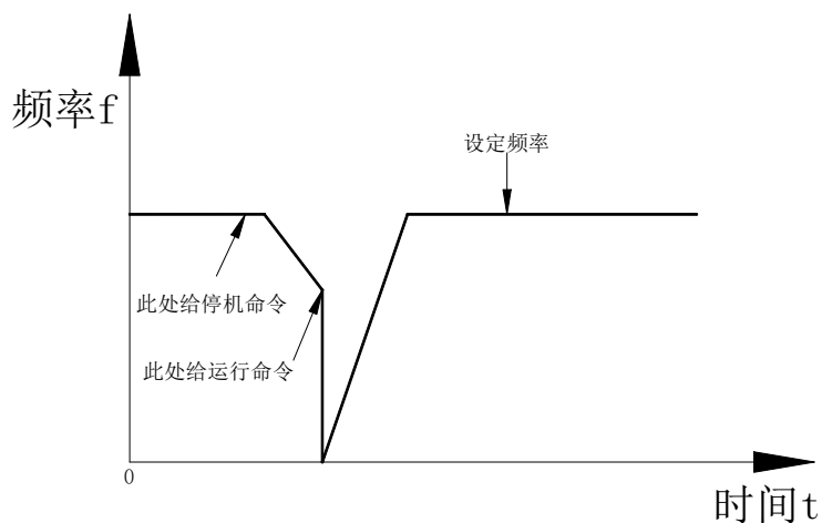
图 10-12 从最小频率做追踪启动
