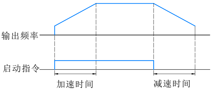
图 10-13 减速停机输出频率曲线
