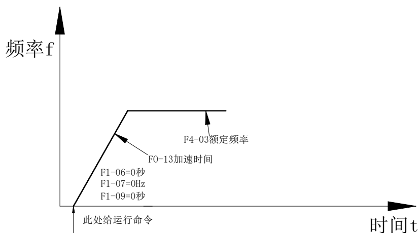
图 10-8 直接启动不带直流制动示意图
