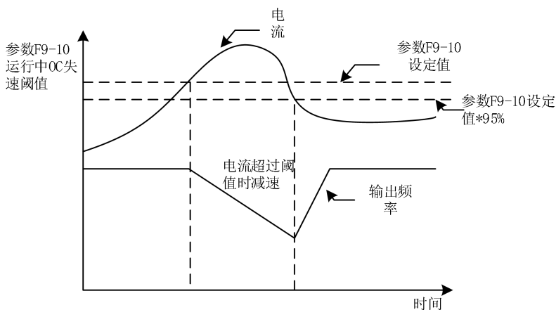
图 9-25 运行中过流失速防止功能
