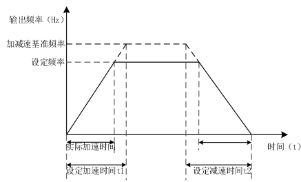
图 9-1 加减速时间
