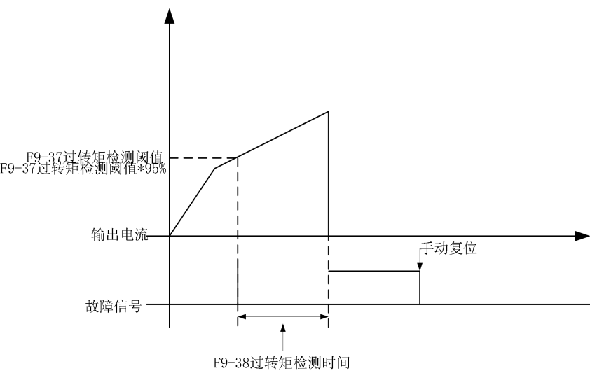
图 9-33 过转矩检测示意图 2
