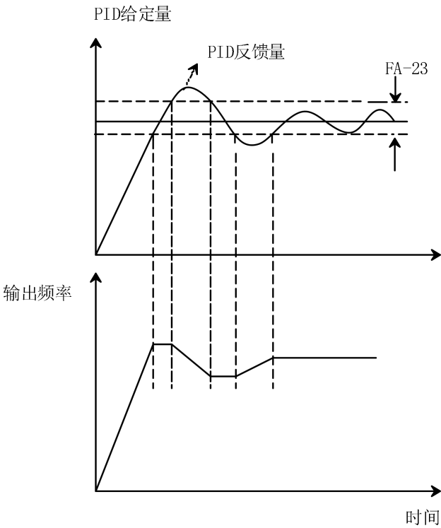
图 9-39 PID 控制偏差极限示意图
