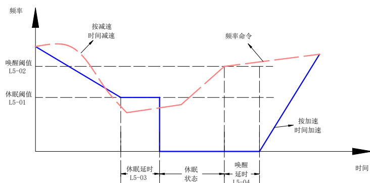
图 10-34 频率命令
