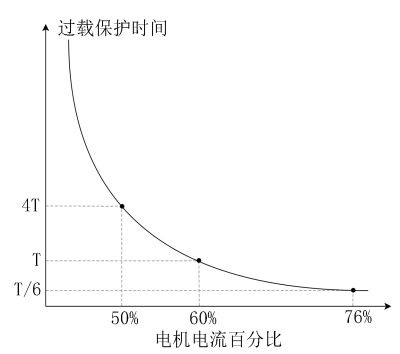
图 9-22 反时限曲线 3
