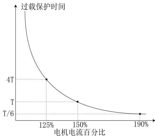
图 9-20 反时限曲线 1
