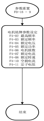
图 10-16 异步电机 VF 调试基本设置
