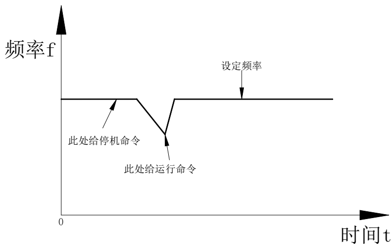
图 10-11 从当前频率做追踪启动
