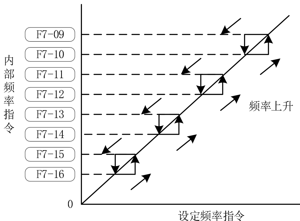
图 10-23 跳频功能
