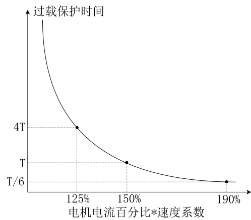
图 9-21 反时限曲线 2
