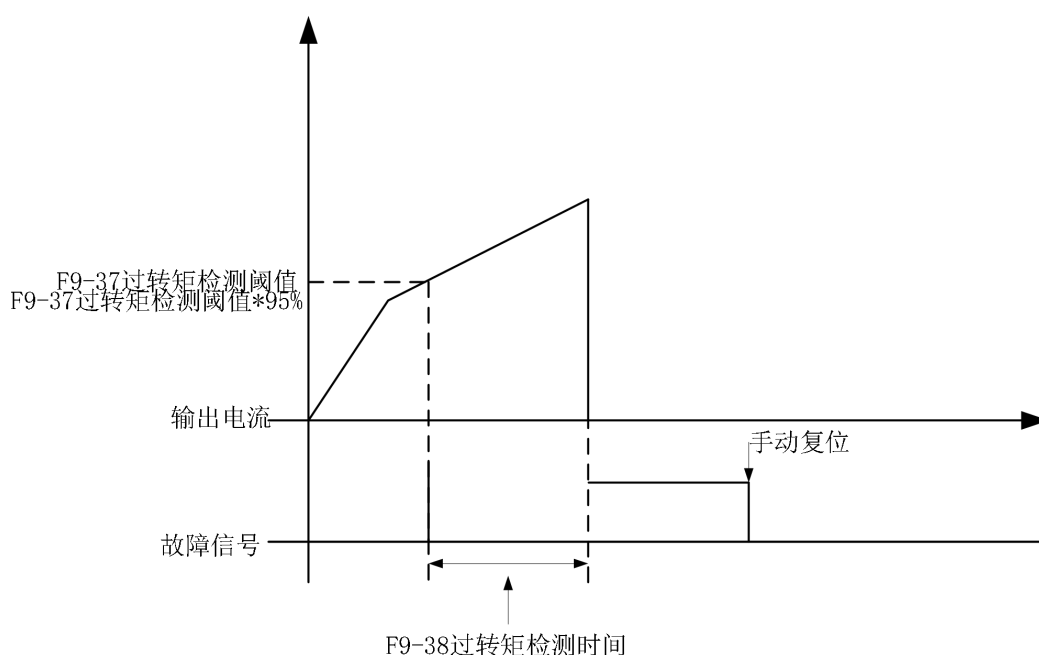
图 10-41 过转矩检测示意图
