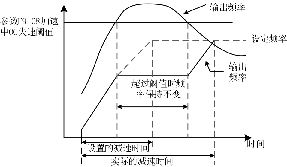
图 10-24 加速中过流失速
