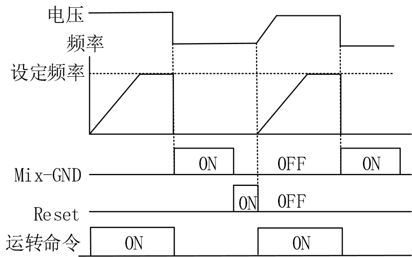
9-12 外部故障自由停车功能
