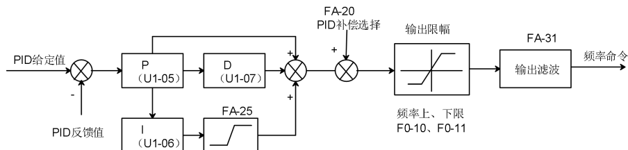
图 10-30 PID 串联控制框图
