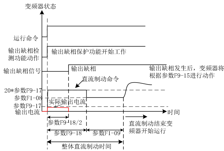
图 9-29 F9-18≠0 且 F1-09≠0，（启动时检测到输出缺相）
