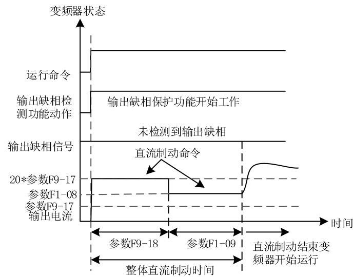
图 10-44 F9-18≠0 且 F1-09≠0（启动时没有检测到输出缺相）
