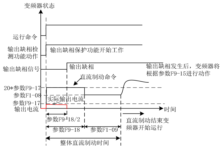
图 10-45 F9-18≠0 且 F1-09≠0（启动时检测到输出缺相）
