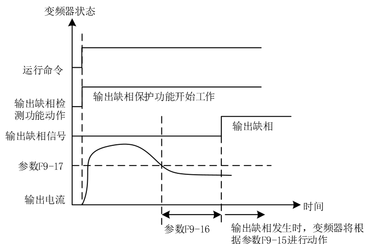
图 9-26 F9-18=0
