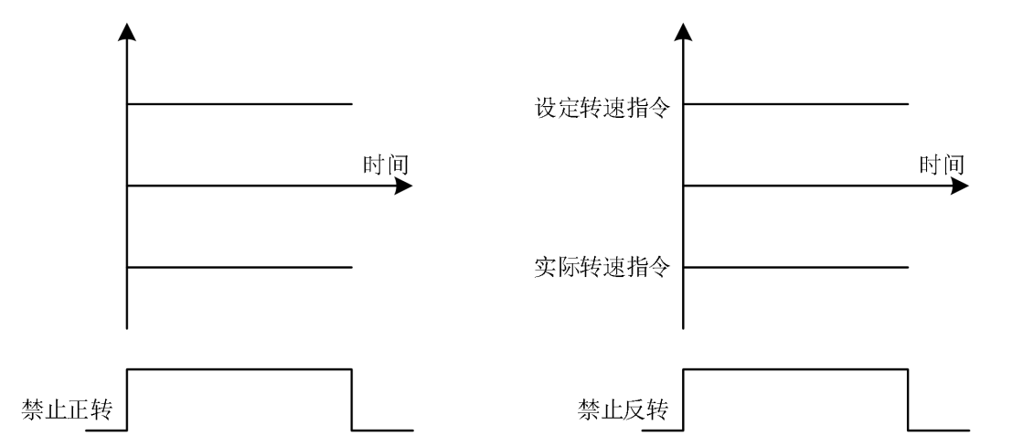
图 10-18 正/反转禁止选择示意图
