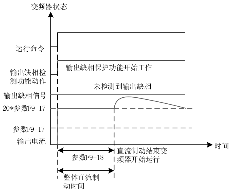
图 10-46 F9-18 \neq 0 且 F1-09=0 (启动时没有检测到输出缺相)
