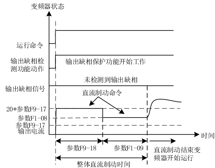
图 9-28 F9-18≠0 且 F1-09≠0（启动时没有检测到输出缺相）
