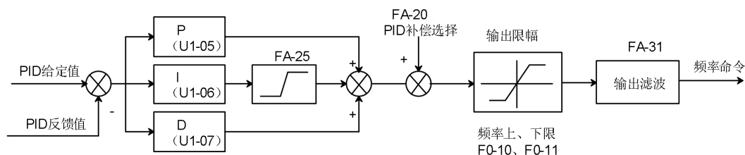
图 10-31 PID 并联控制框图
