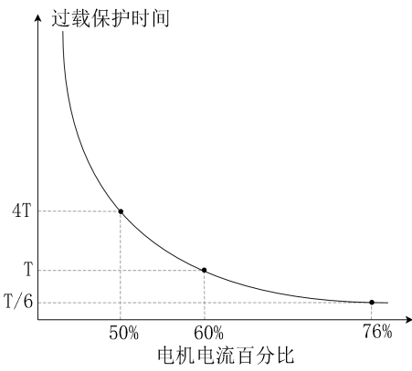
图 10-39 反时限曲线 3
