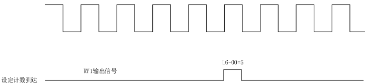
图 9-44 最终计数值设定示意图
