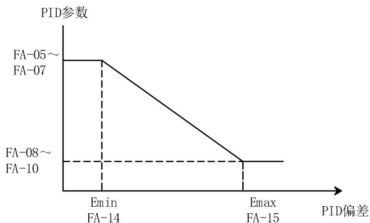
图 9-38 PI 参数调节示意图
